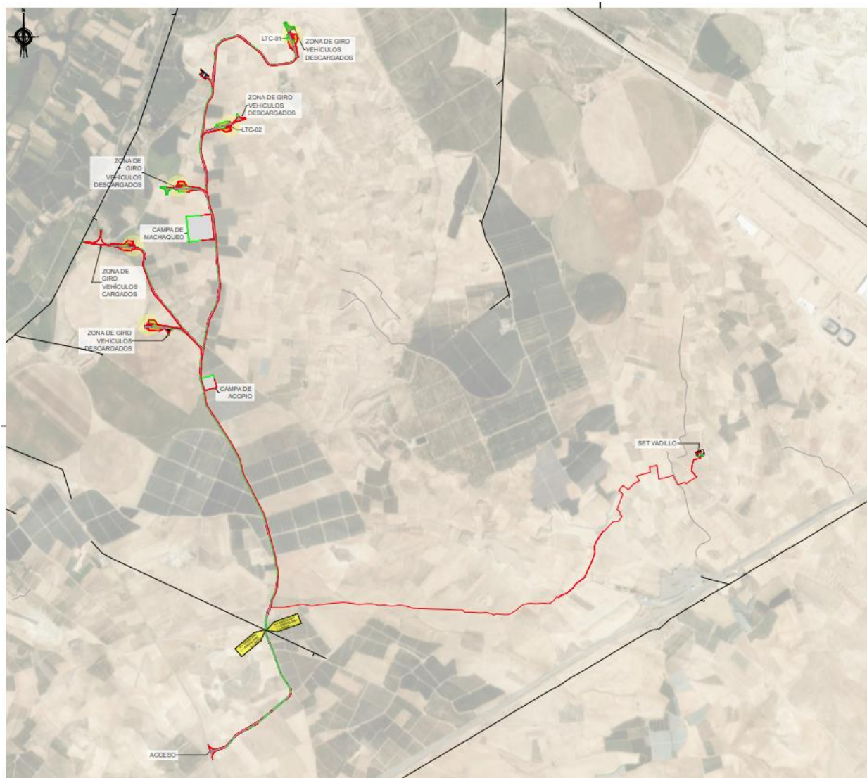
Imagen 21: Imagen general de las líneas eléctricas de Endesa afectadas
