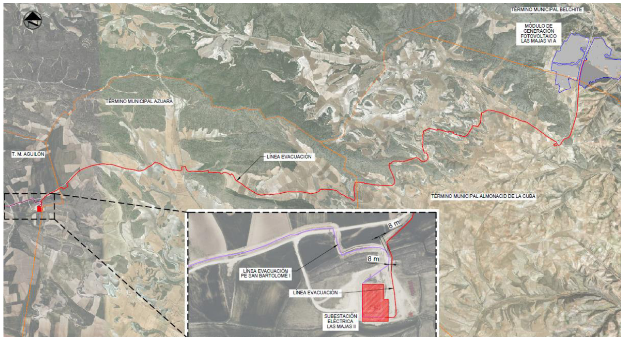
Ilustración 4: Paralelismo de línea de evacuación subterránea MT 30 kV con zanja de parque eólico SAN BARTOLOMÉ I
