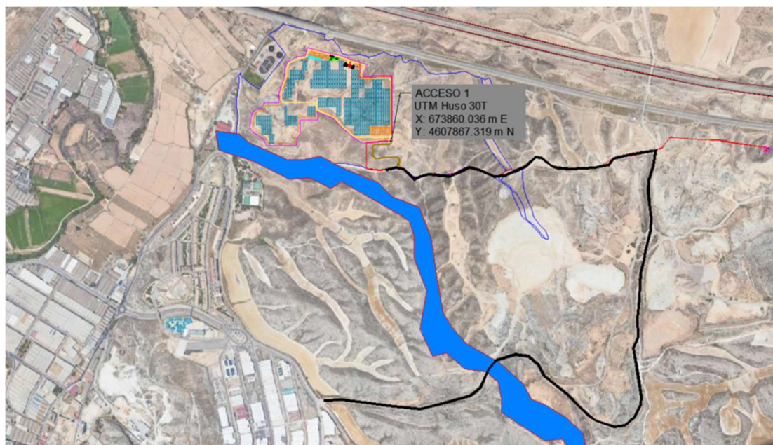
Figura 4: Acceso al Parque Solar FV.
