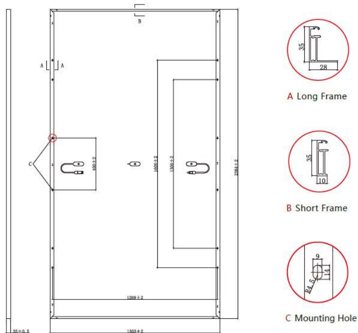
Figura 27: Dimensiones del Módulo.
