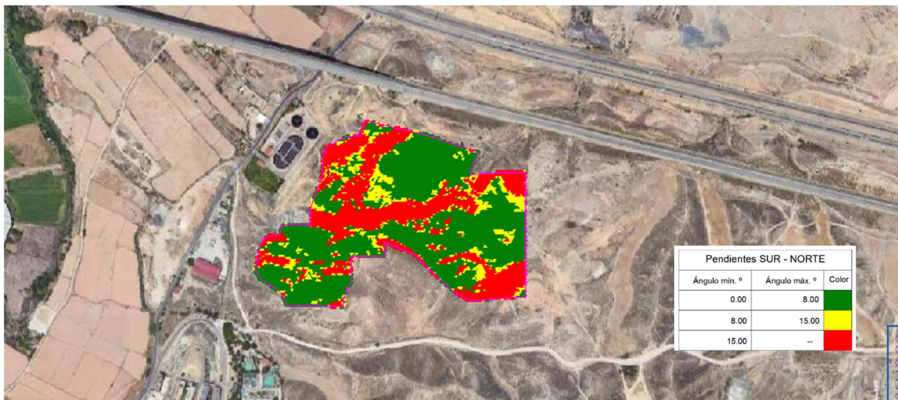
Figura 6: Pendientes Sur – Norte.
