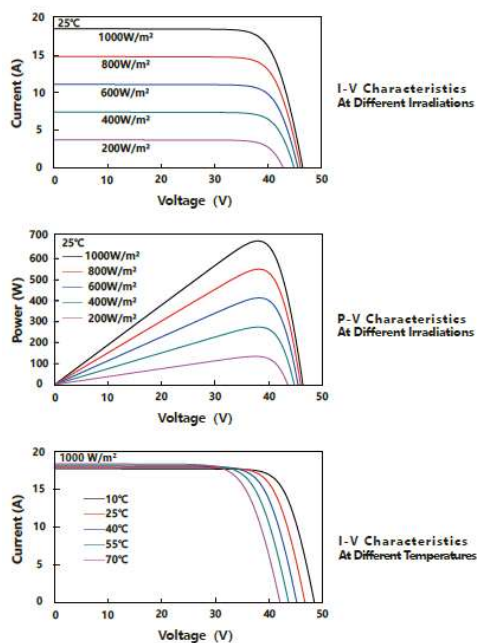
Figura 28: Curvas Características JW-HD132N.
