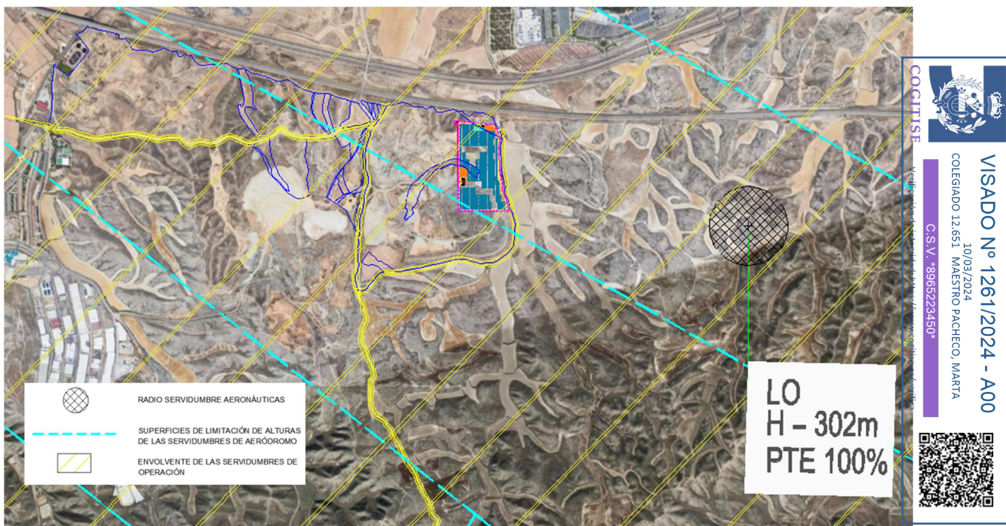
Figura 24: Servidumbres aeronáuticas.
