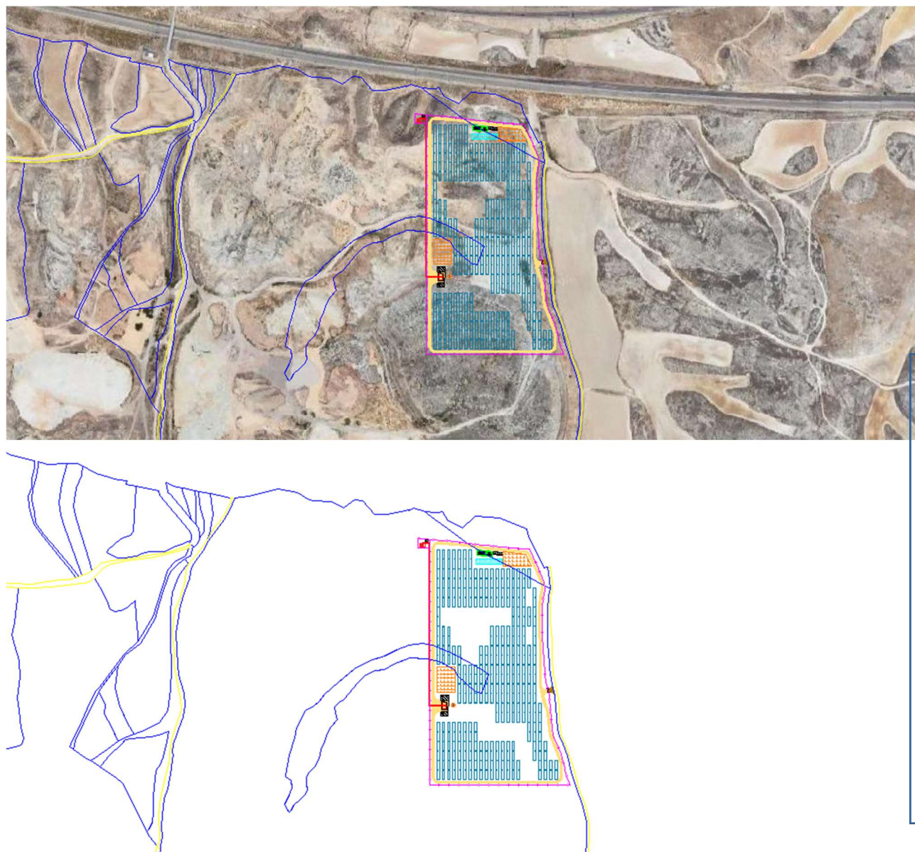
Figura 26: Instalación FV.
