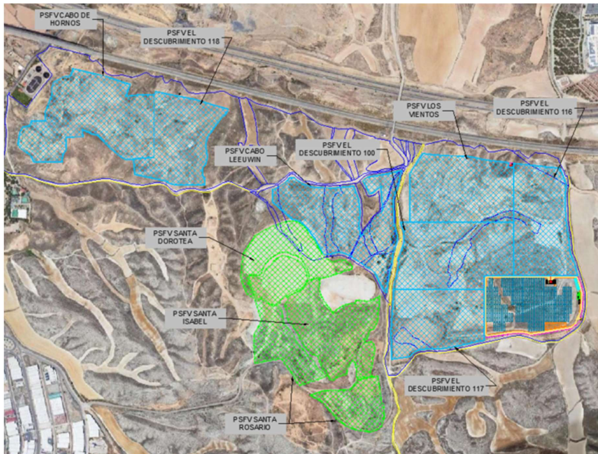
Figura 1: Parques Fotovoltaicos.
