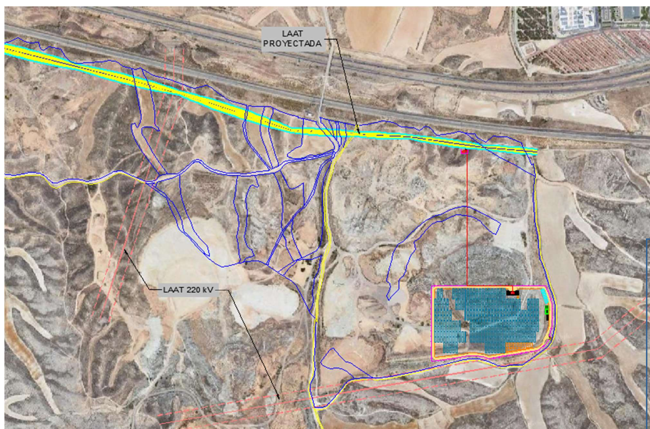
Figura 18: Líneas eléctricas.
