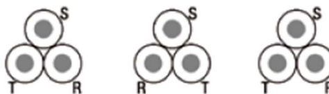
Figura 31: Colocación de cables en tresbolillo.
