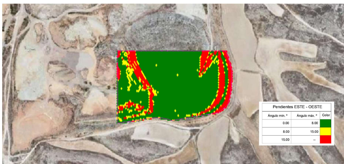
Figura 7: Pendientes Este – Oeste.
