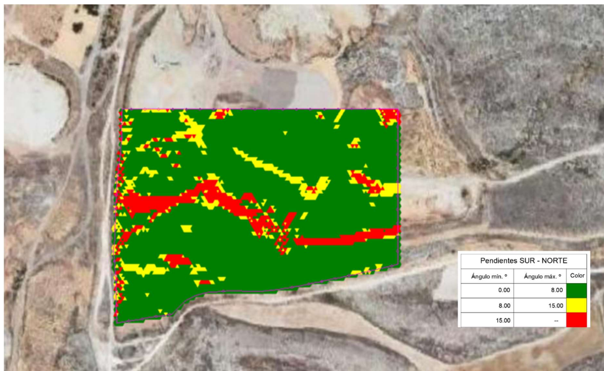
Figura 6: Pendientes Sur – Norte.
