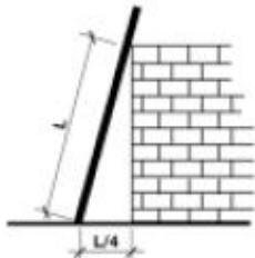
INCLINACIÓN RECOMENDADA
