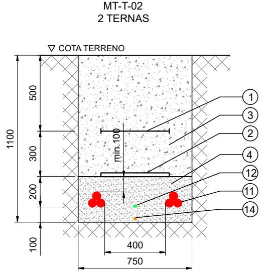
CRUCE SECCIÓN TIPO ZANJA CON AFECCIÓN 01
