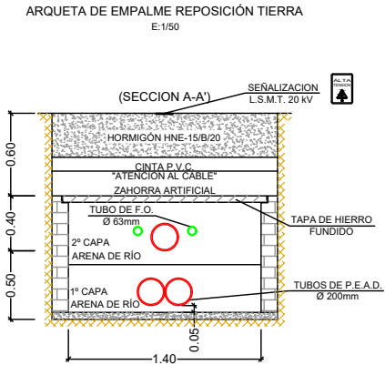
DETALLES ARQUETAS DE EMPALME PARA ZANJA TIPO 2 3 Tubo 200 Ø
