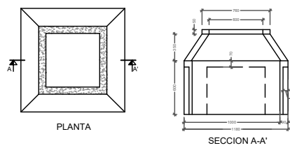
MARCO Y TAPA TIPO M3-T3 CALZADA - ARQUETA PREFABRICADA (S/E)
