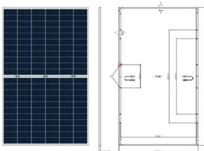
Figura 8: Dimensiones del Módulo
