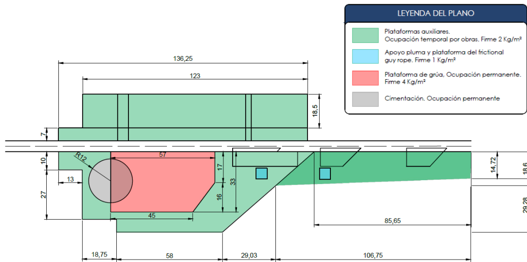
Ilustración 7. Plataforma tipo
