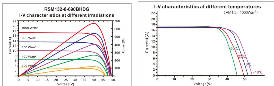
Ilustración 6. Curvas características
