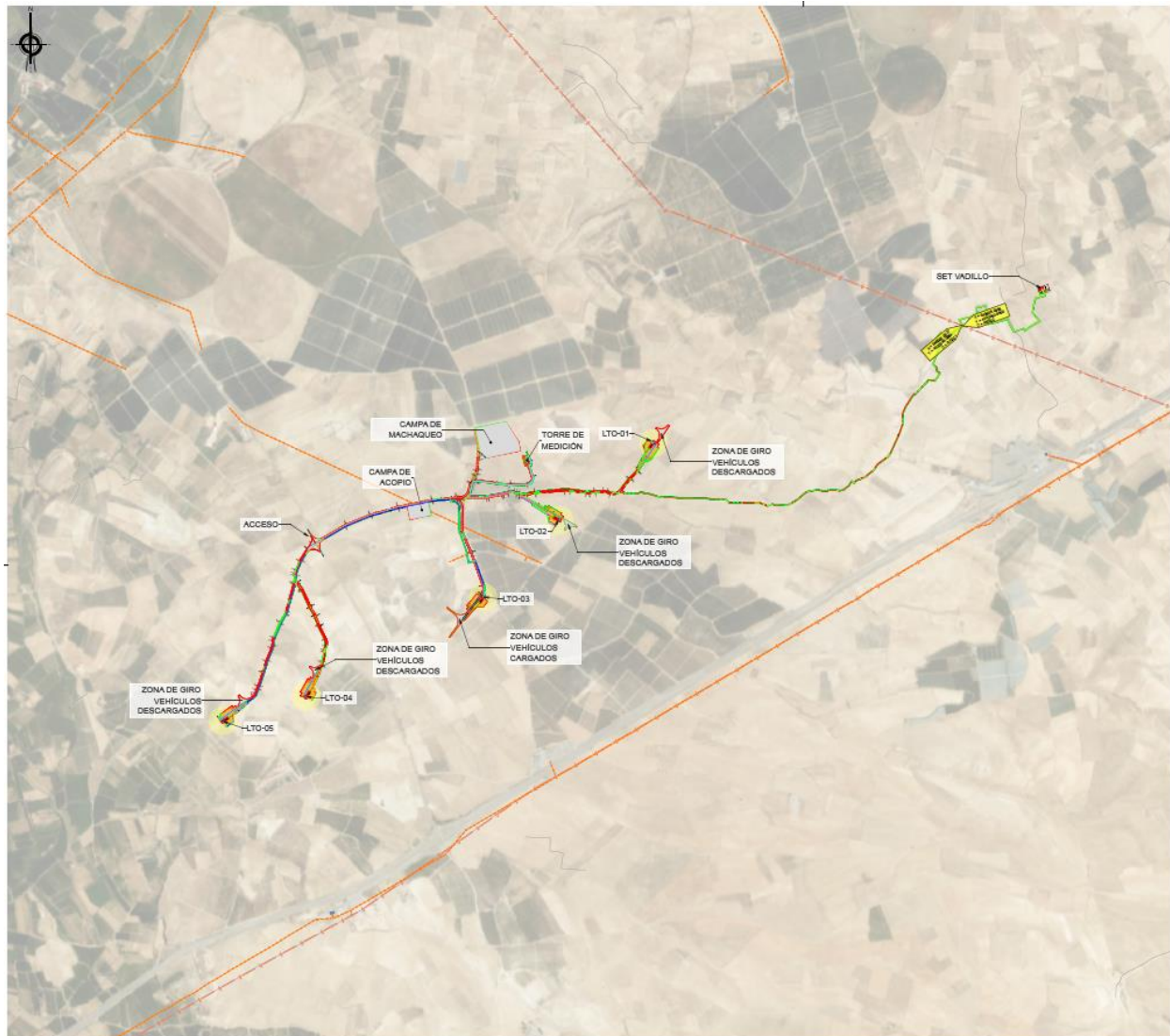
Imagen 20: Vista aérea de las líneas aéreas de media/alta tensión cercanas al parque eólico LITIO
