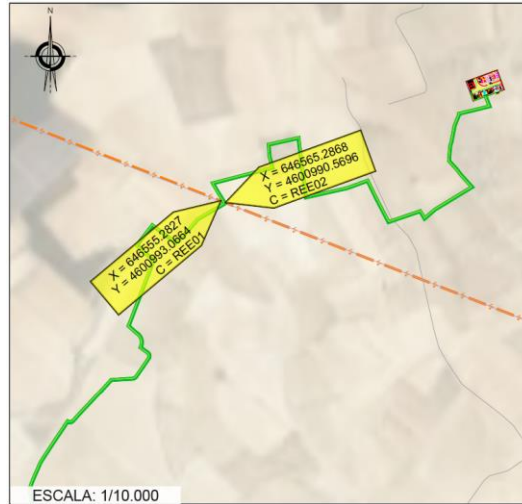
Imagen 21: Vista en detalle de los cruces de línea aérea de alta tensión (220 kV) con la línea de evacuación de media tensión subterránea del parque eólico LITIO
