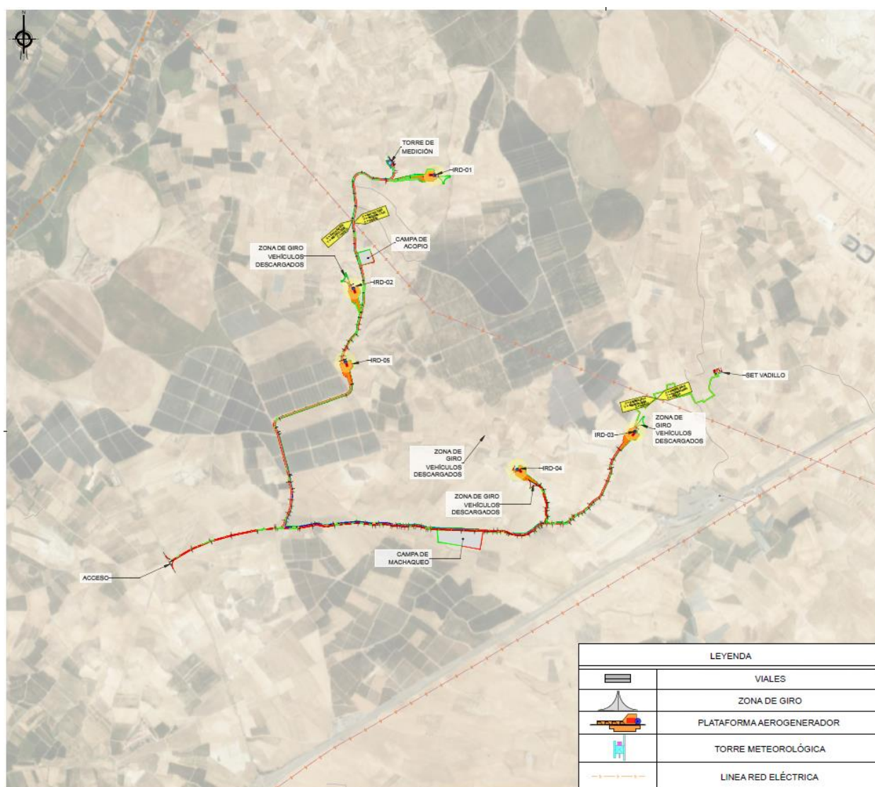
Imagen 21: Vista aérea de las líneas aéreas de media/alta tensión cercanas al parque eólico IRIDIO
