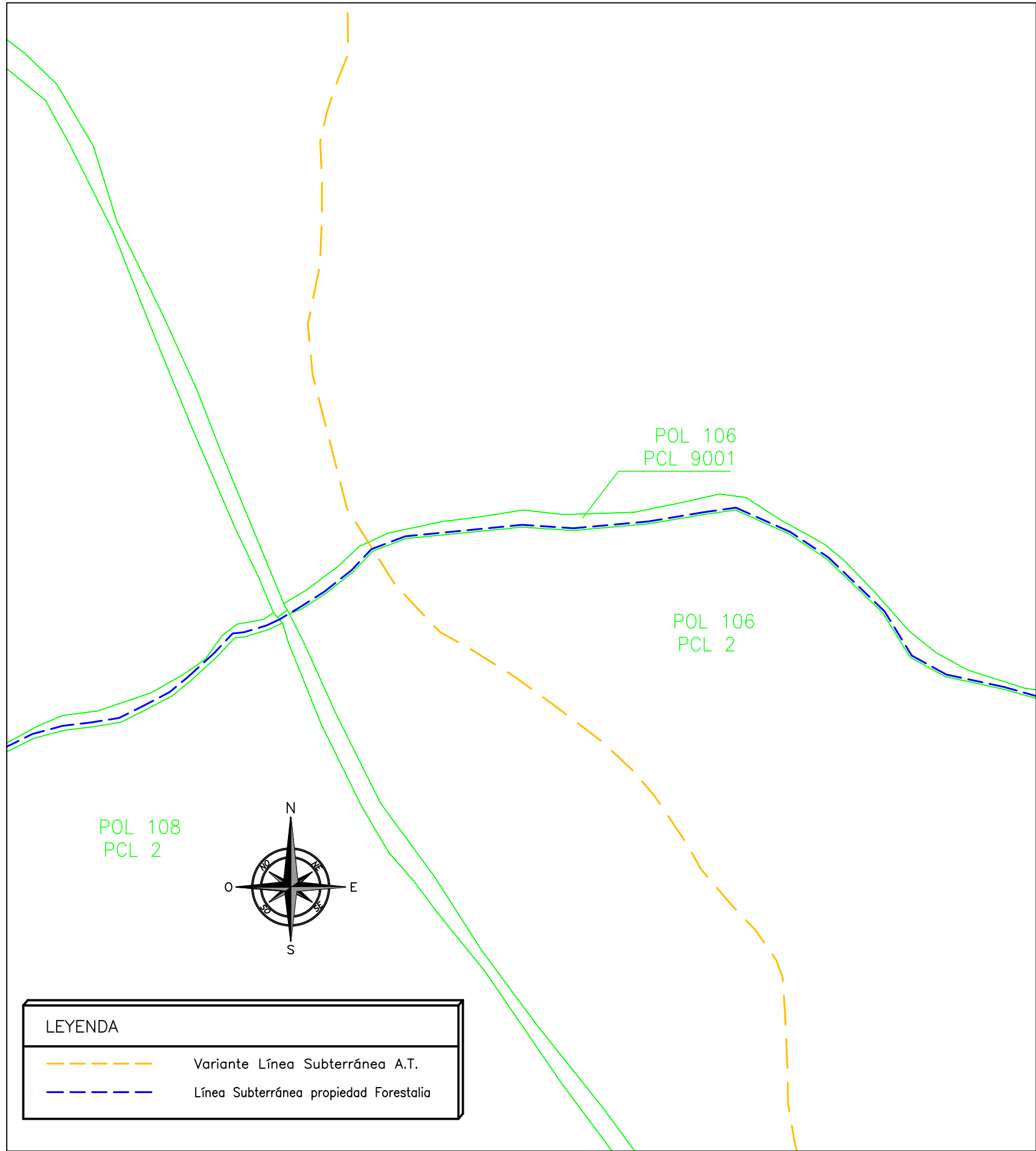
PLANTA ESCALA 1:2.000
