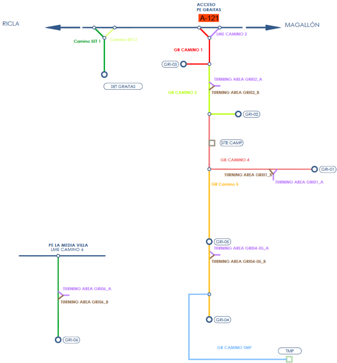
Ilustración 6. Viales interiores del PE
