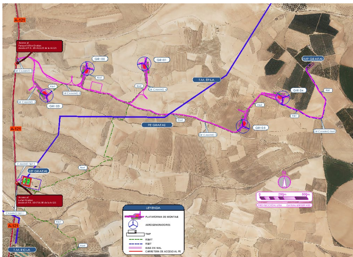
Ilustración 3. Cruzamiento del camino 5 y de la RSMT con línea de E-Distribución Redes Digitales
