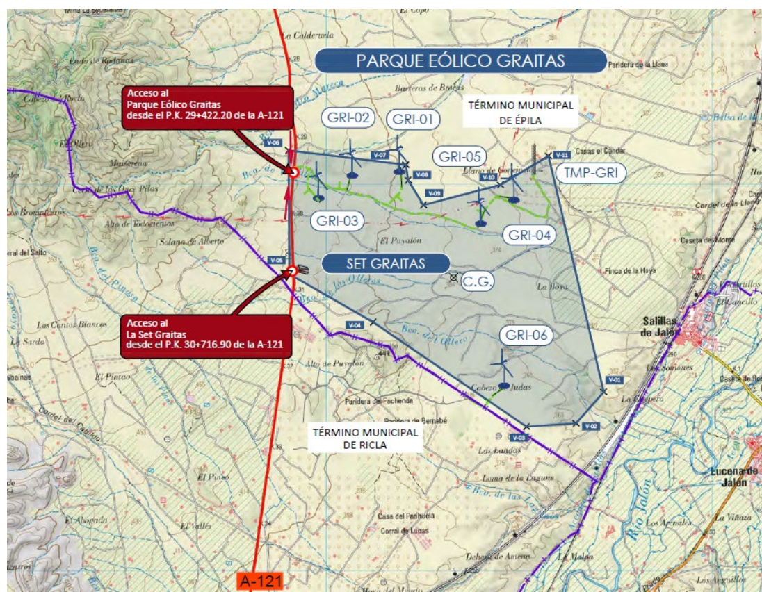
Ilustración 5. Accesos al PE
