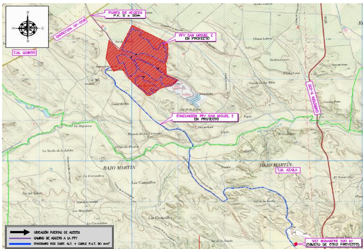
Ilustración 2: Accesos a la planta FV
