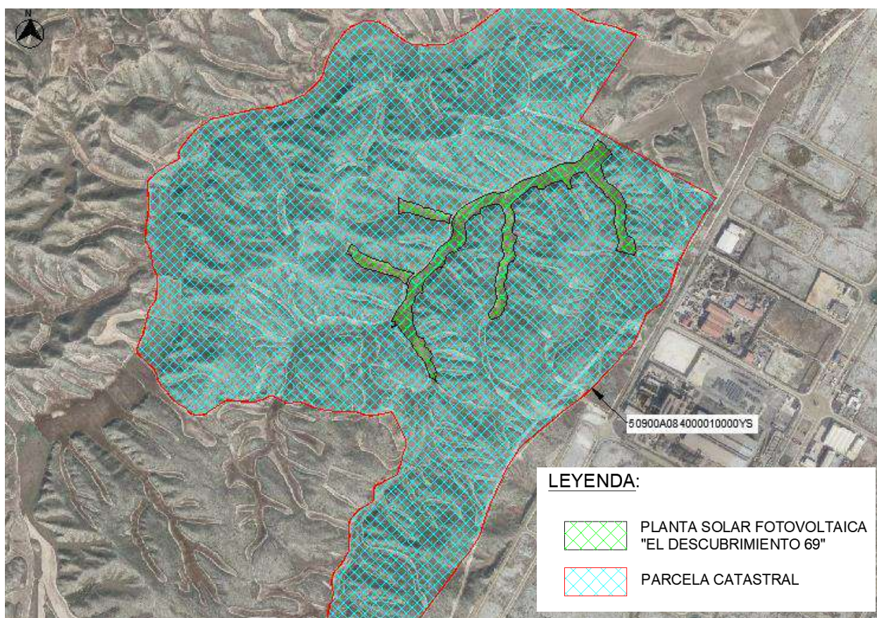
Figura 2: Área Disponible, Vallado Perimetral del Parque Solar
