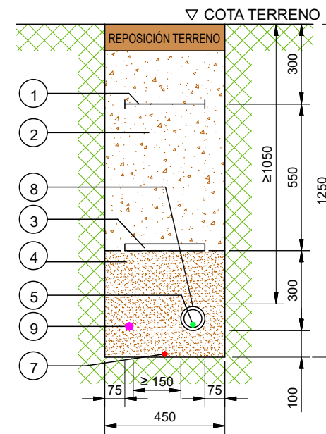
SECCION ZANJA TIPO EN TIERRA 1 LINEA DE B.T.
