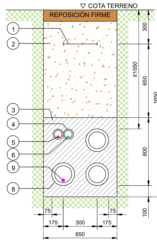
SECCION ZANJA TIPO EN CRUCE DE CAMINO 1 TERNA DE B.T.
