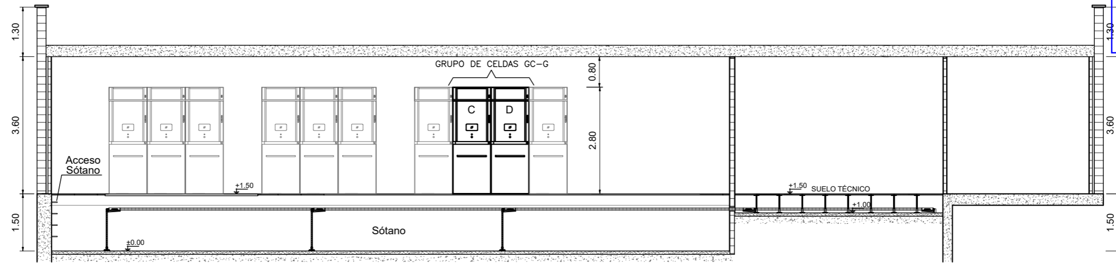
SECCIÓN A-A'
