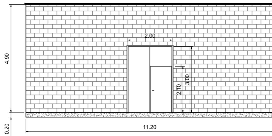
ALZADO B
