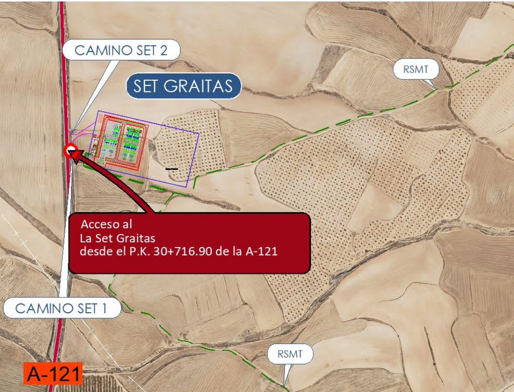
Ilustración 4. Afección de Entronque y zona de afección de la zanja RSMT en el P.K. 30+716.90 de la A-121
