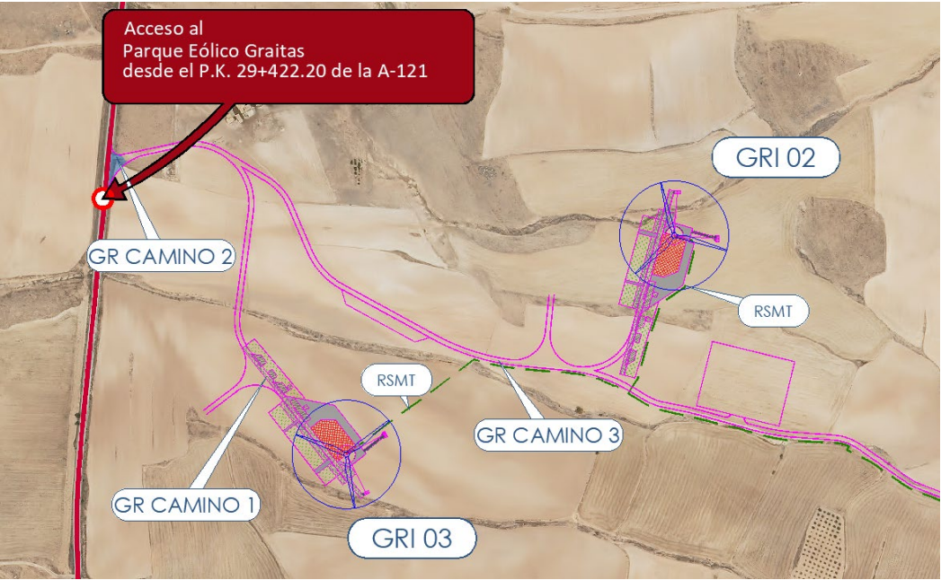
Ilustración 3. Afección de Entronque P.K. 29+422.20 de la A-121
