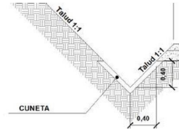
Imagen 14: Cuneta tipo
