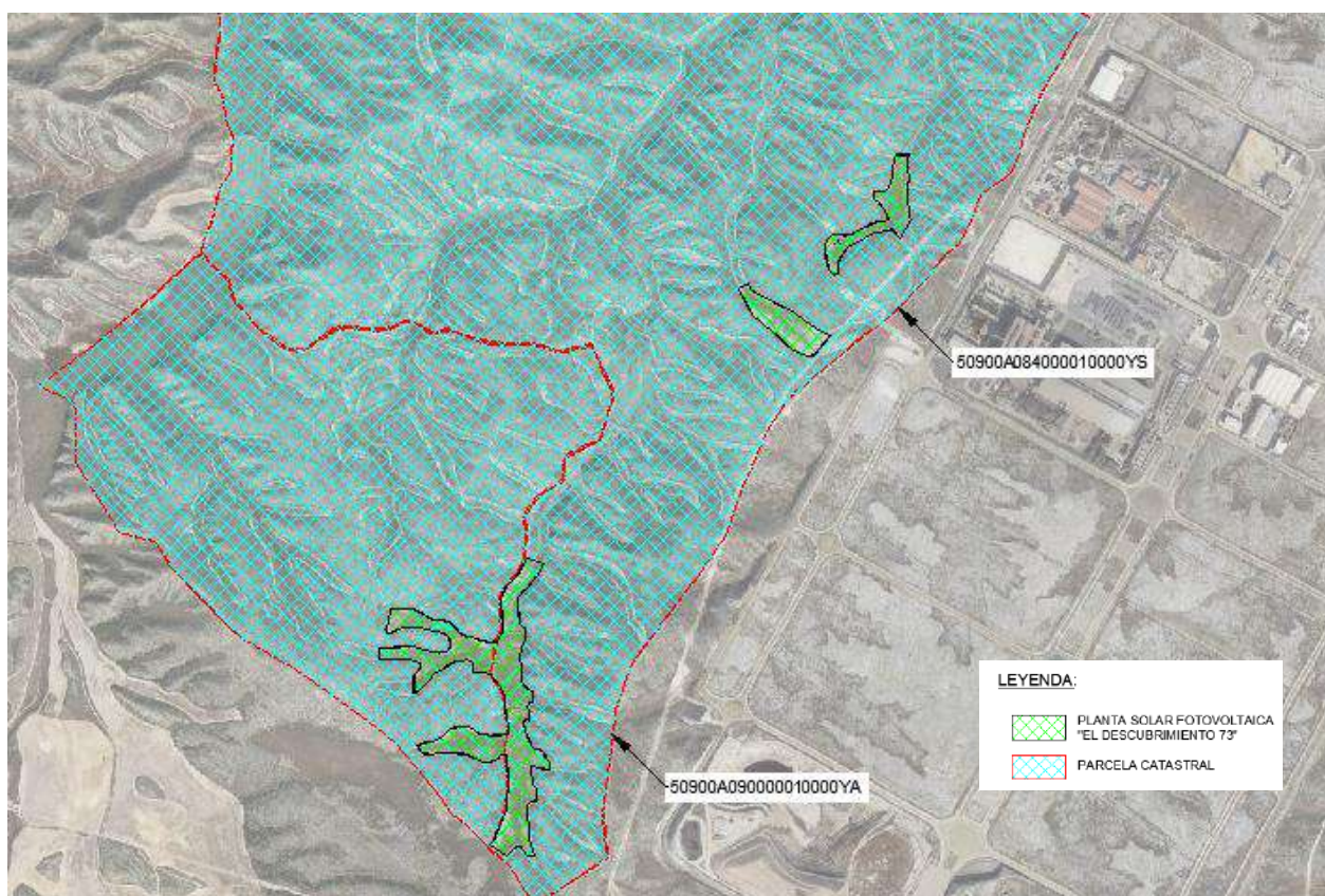
Figura 2: Área Disponible, Vallado Perimetral del Parque Solar
