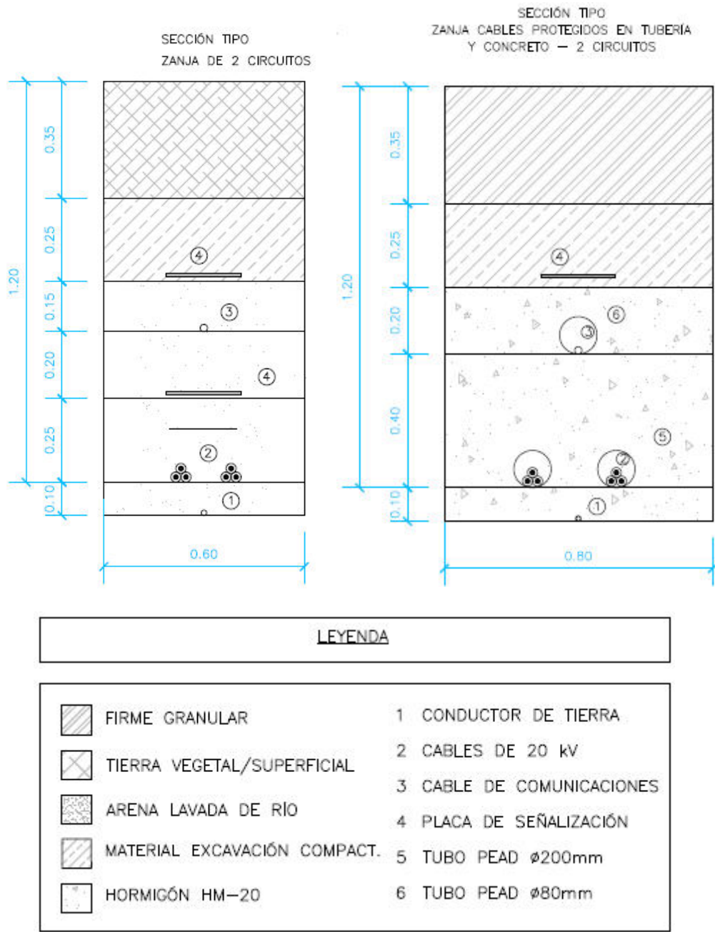
Ilustración 1. Sección tipo zanja de 2 circuitos libre de cruces (izquierda)/ Sección tipo zanja de 2 circuitos cruces viales(derecha)
