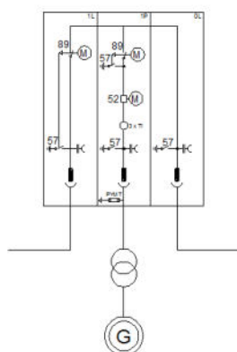
Imagen 9. Esquema unifilar Centro de Transformación tipo II.
