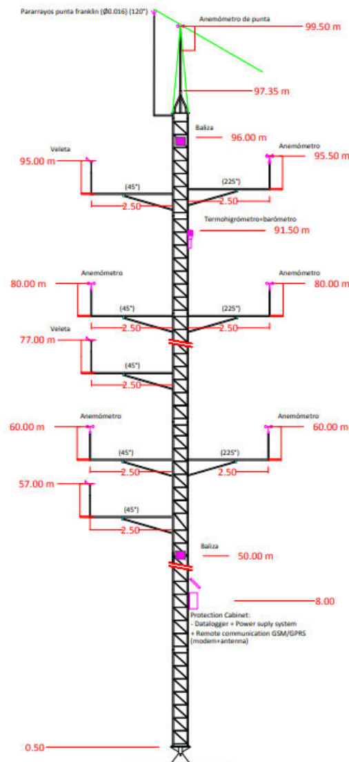
Imagen 2. Esquema conceptual de la torre de medición
