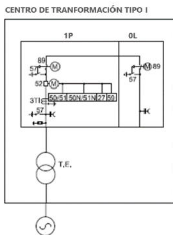
Imagen 8. Esquema unifilar Centro de Transformación tipo I.
