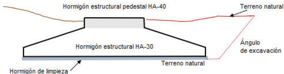
Imagen 4. Esquema dimensional de zapata (sin escala)
