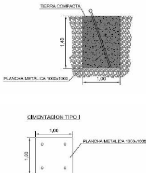
Imagen 5. Detalle cimentación torre de medición
