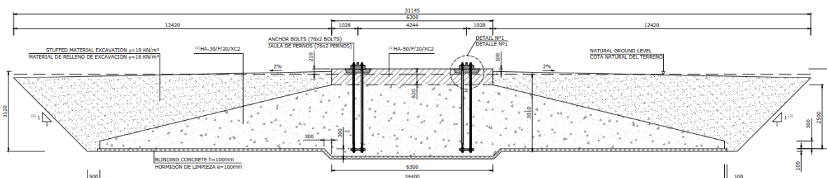
Figura 9: Cimentación del aerogenerador GE158 para una altura de buje de 120,9 m.
