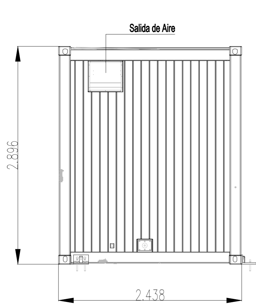
Vista Derecha
