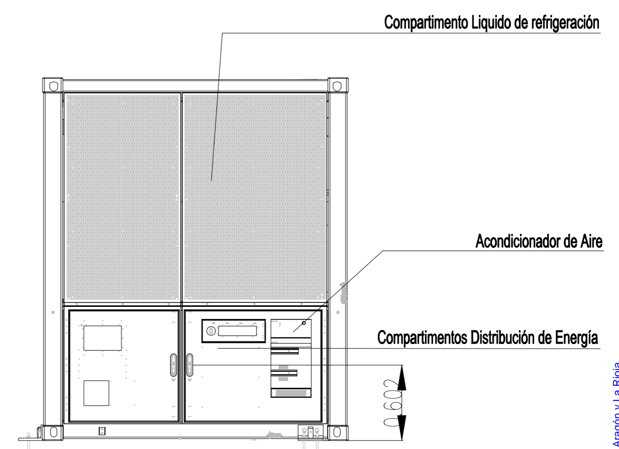
Vista Izquierda
