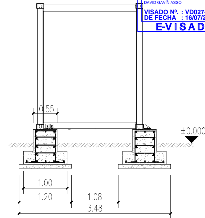
SECCIÓN B-B
