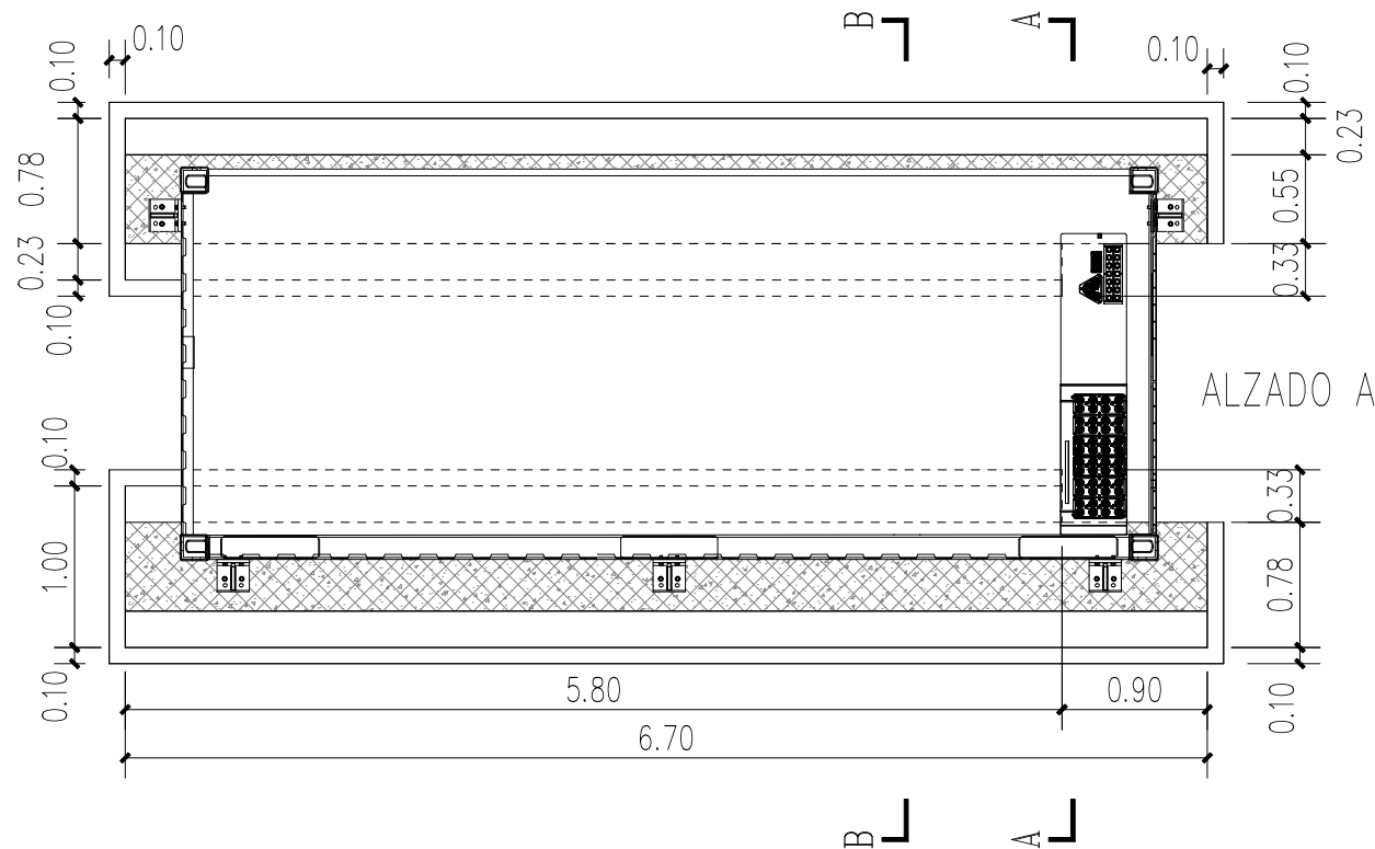
DISEÑO CIMENTACIÓN
