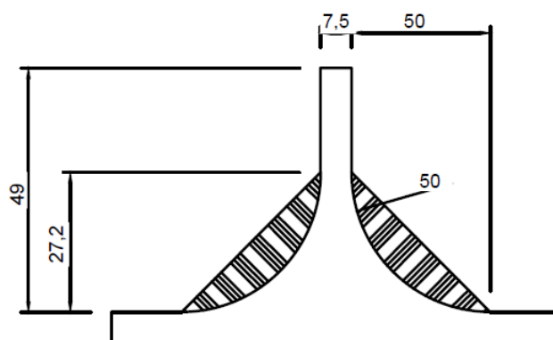
Ilustración 8. Detalle de áreas de giro de camión
