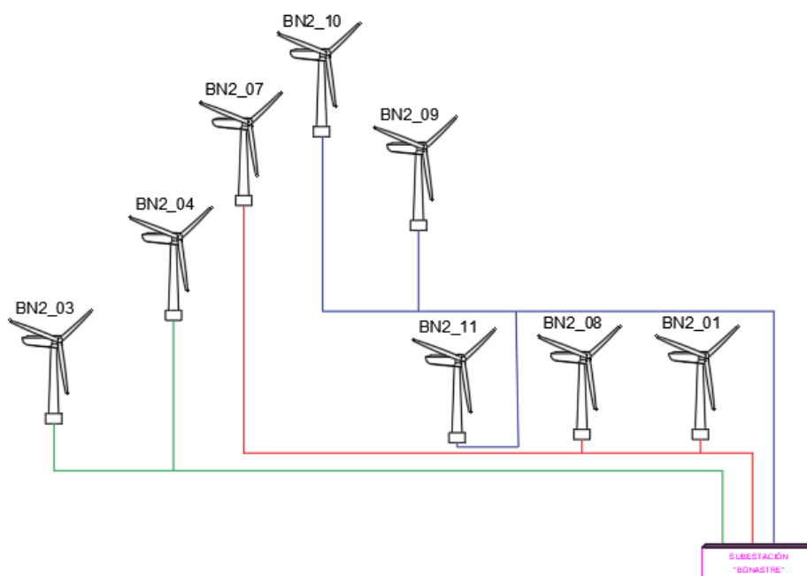
Ilustración 3. Esquema de red eléctrica
