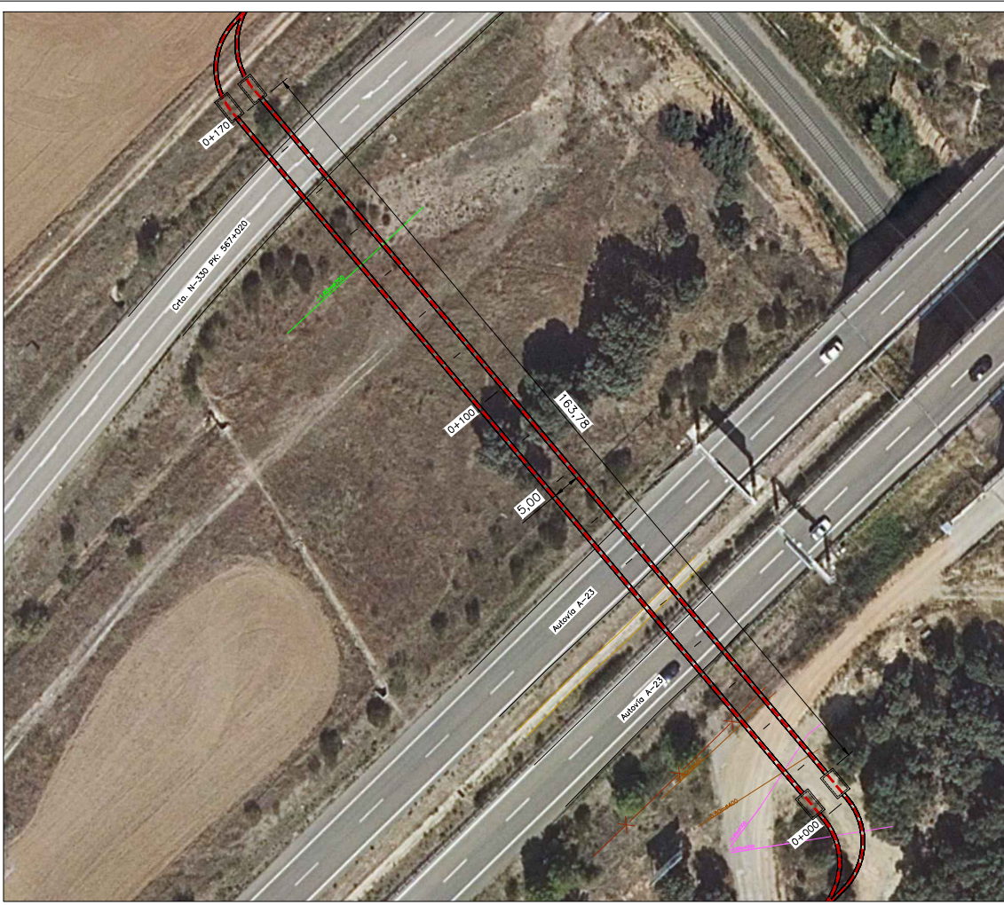
PLANTA Escala 1:1.250
