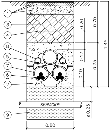
SECCIÓN TIPO PARA CRUZAMIENTO CON SERVICIOS CABLES ELÉCTRICOS
