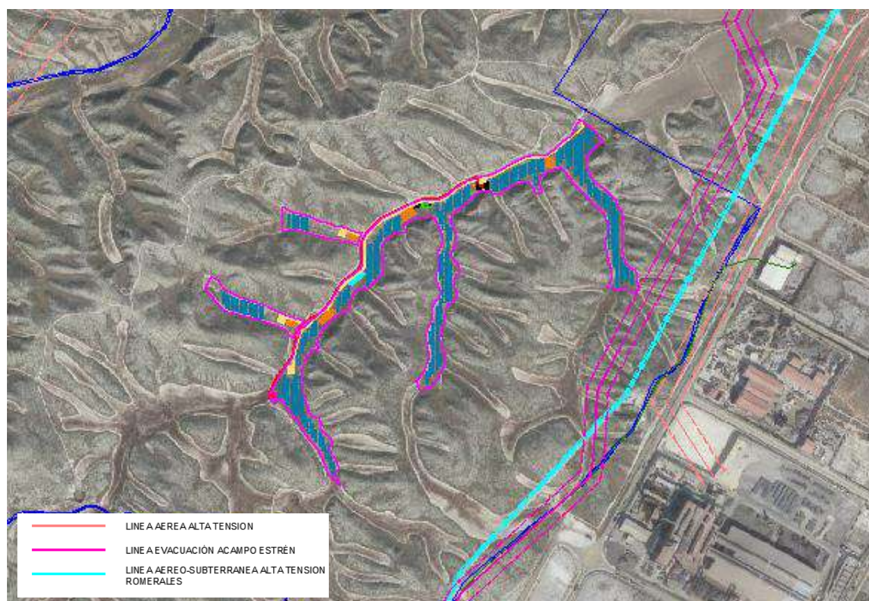
Figura 10: Mapa de líneas eléctricas.
