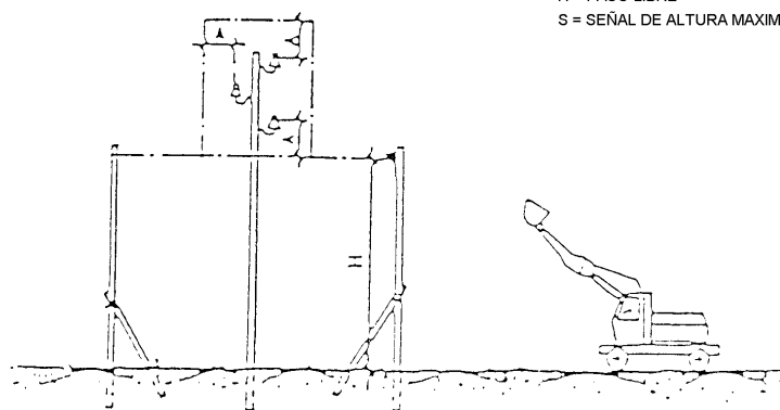
DETALLE - 2
