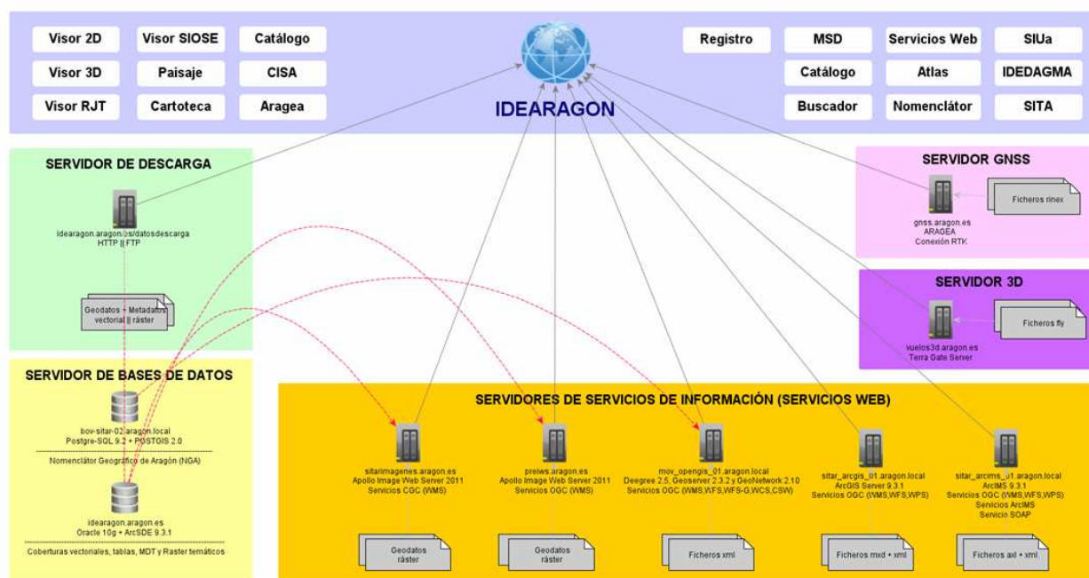
Figura Nº 5. Arquitectura DE IDEARAGON. Año 2015.
