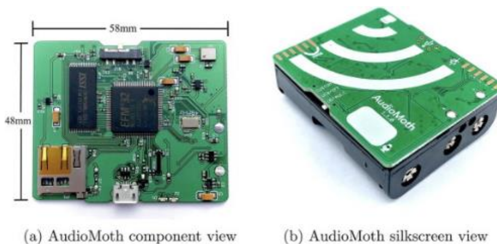
Figura 20. Audiomoth: vista del interior (a) y del exterior (b). Fuente: Hill et al. (2019).
