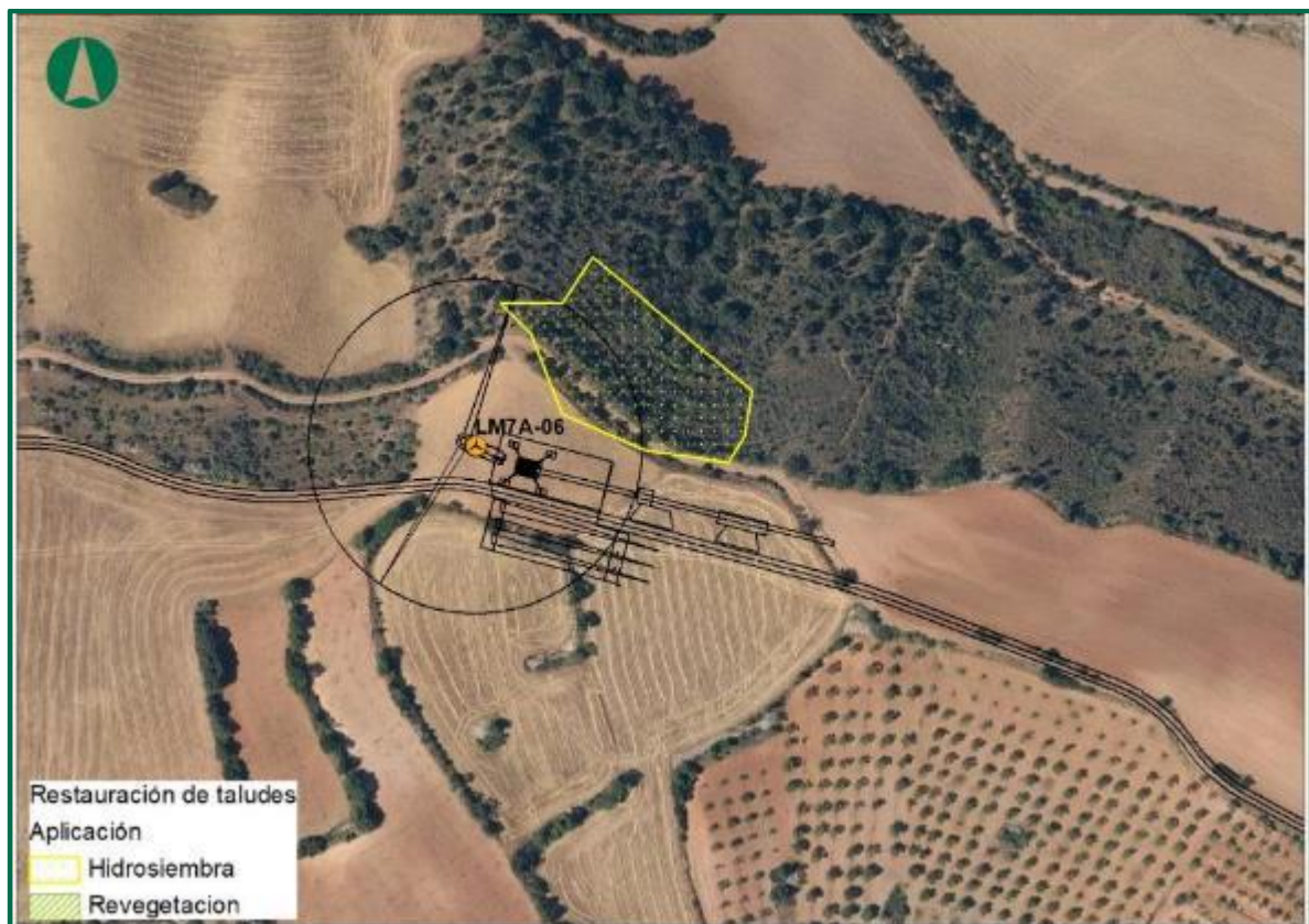
Figura 43. Ubicación del talud a restaurar en el clúster Aguasvivas.
