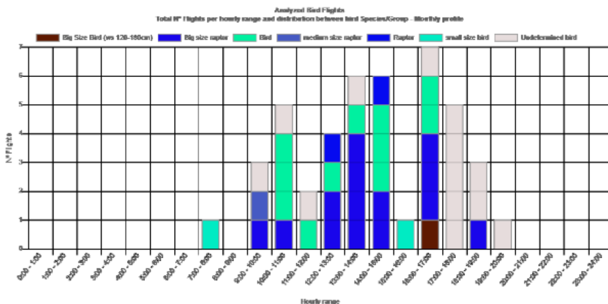
Figura 62. Vuelos analizados por especie, perfil cuatrimestral por horas. WTG LM7E-05 Fuente: DtBird.
