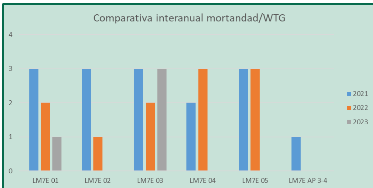
Figura 33. Mortalidad interanual para el primer cuatrimestre por posición, en el PE Las Majas VII E.
