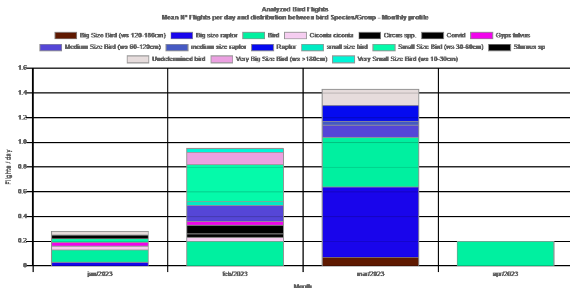
Figura 61. Vuelos analizados por especie, perfil cuatrimestral por horas. WTG LM7E-04 Fuente: DtBird.
