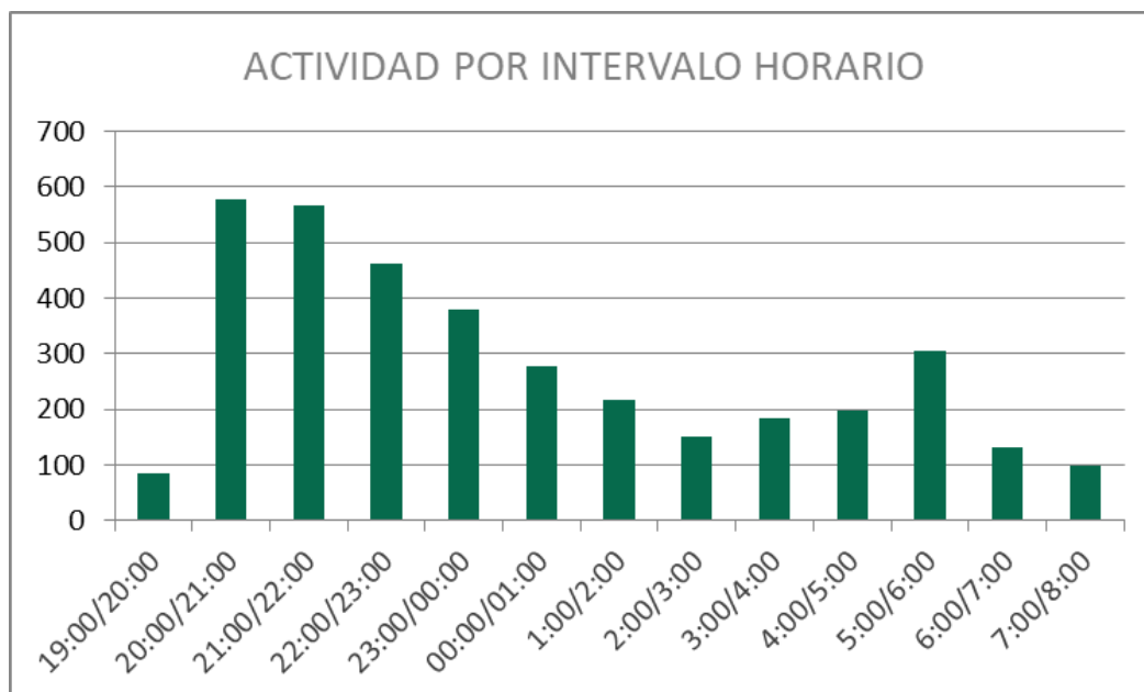
Figura 22. Registros totales en función de la hora.
