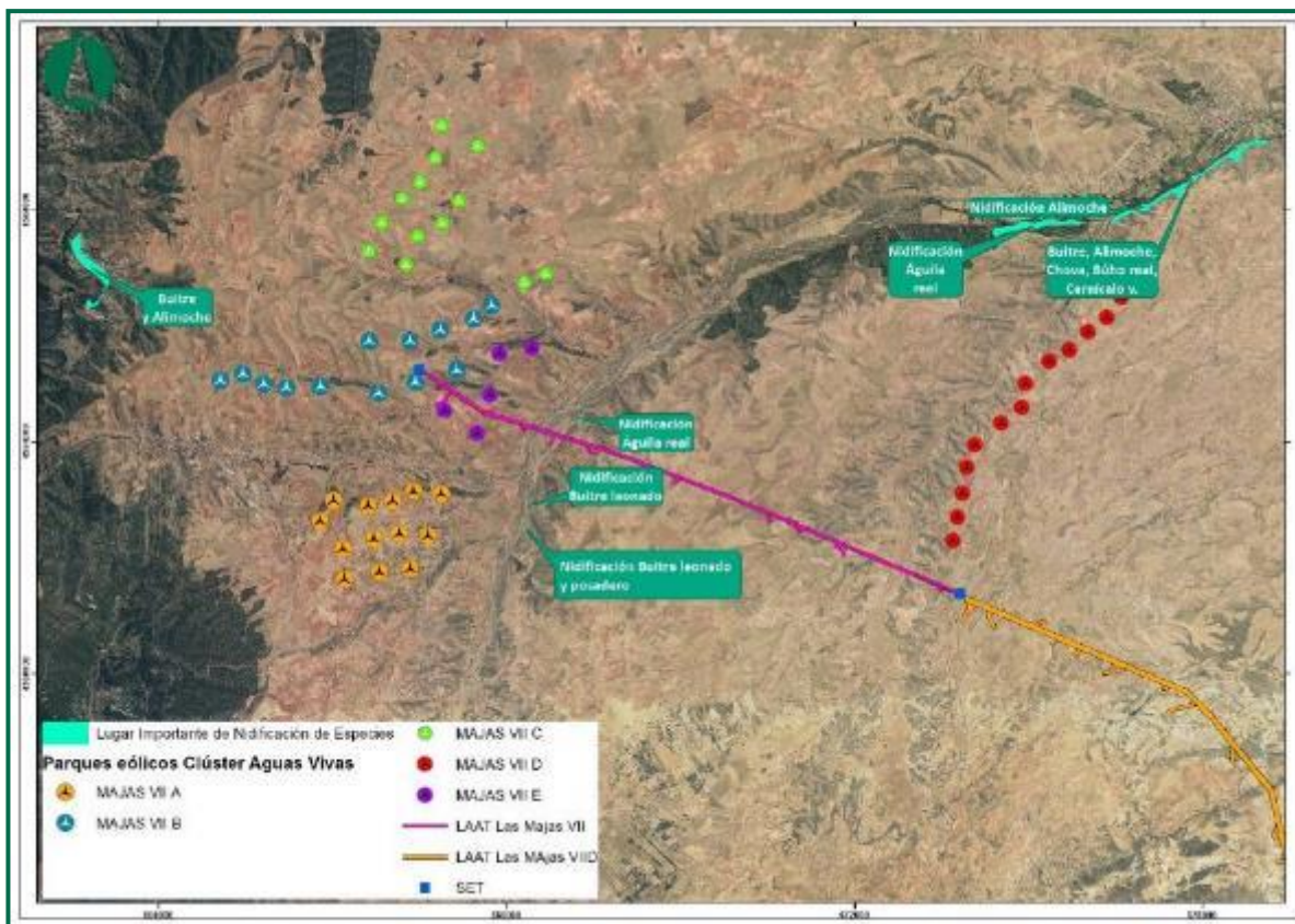
Figura 14. Situación de zonas de fauna establecidas como lugar importante de nidificación de especies.
