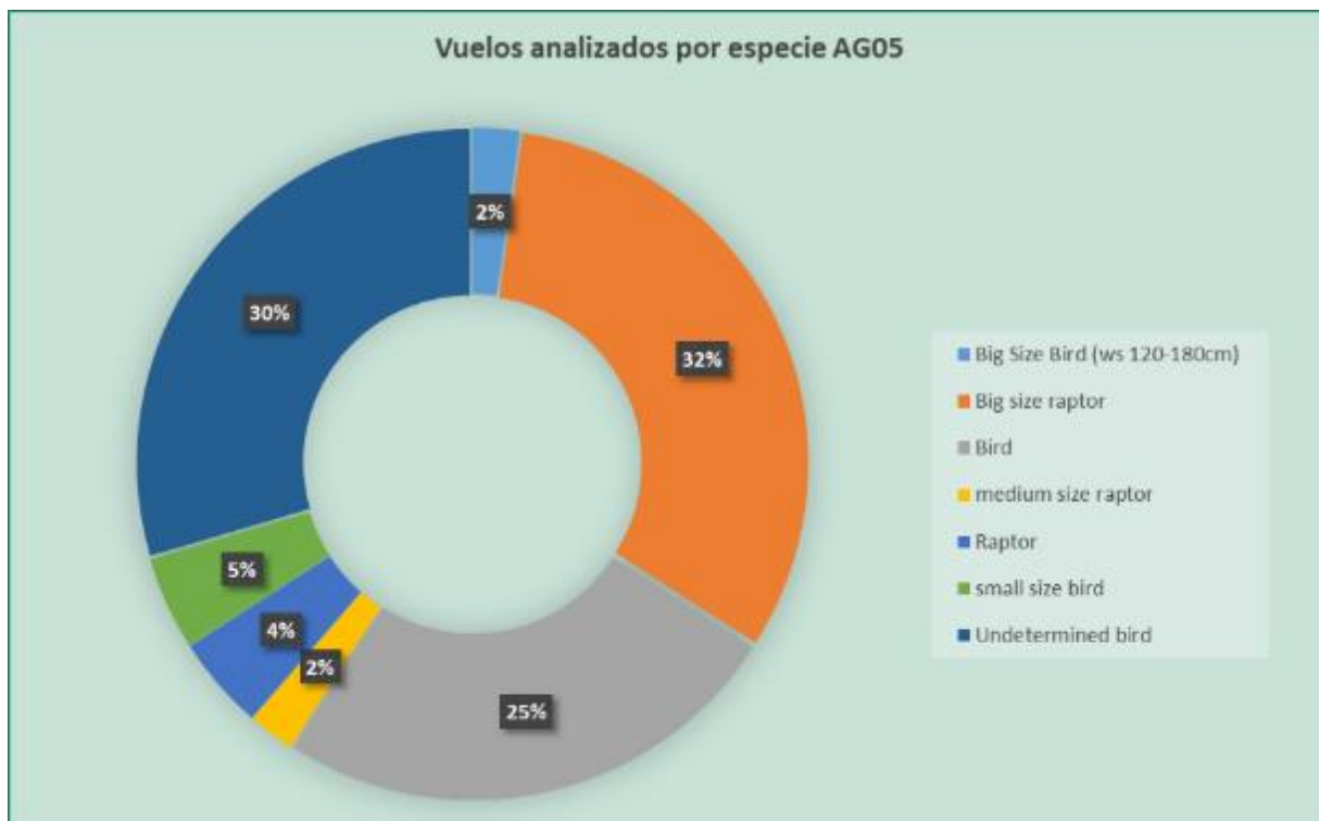
Figura 60. Porcentaje de vuelos por especie/grupo AG05.
