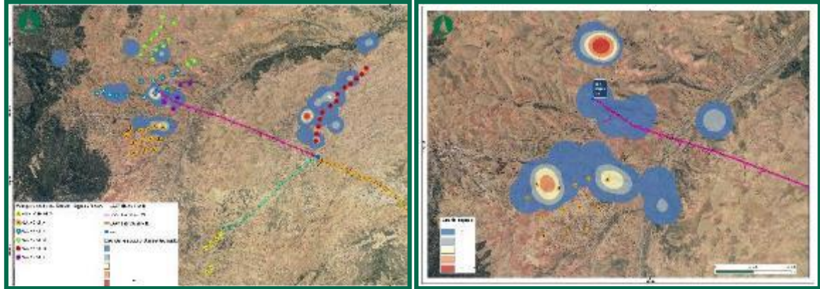
Figura 11. Intensidad del uso del espacio de buitre leonado ( Gyps fulvus ), 1 er cuatrimestre 2021.
