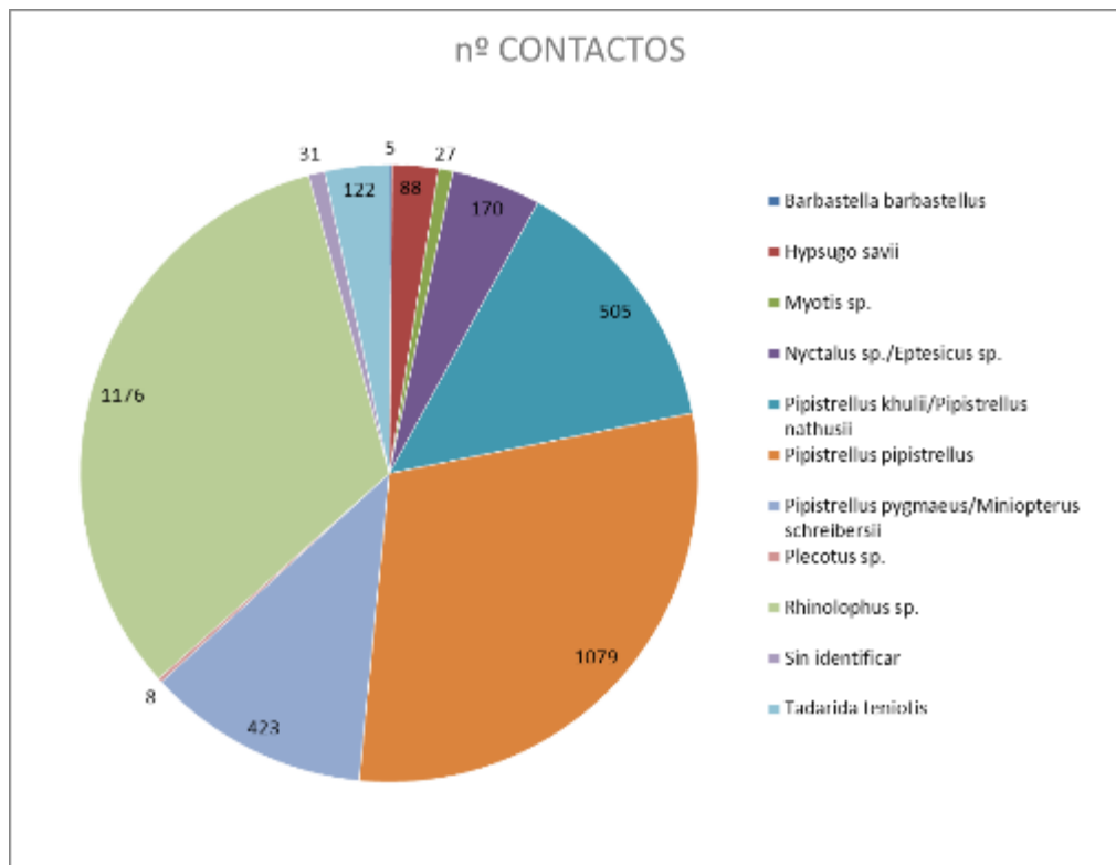
Figura 20. Registros totales de las diferentes especies identificadas.
