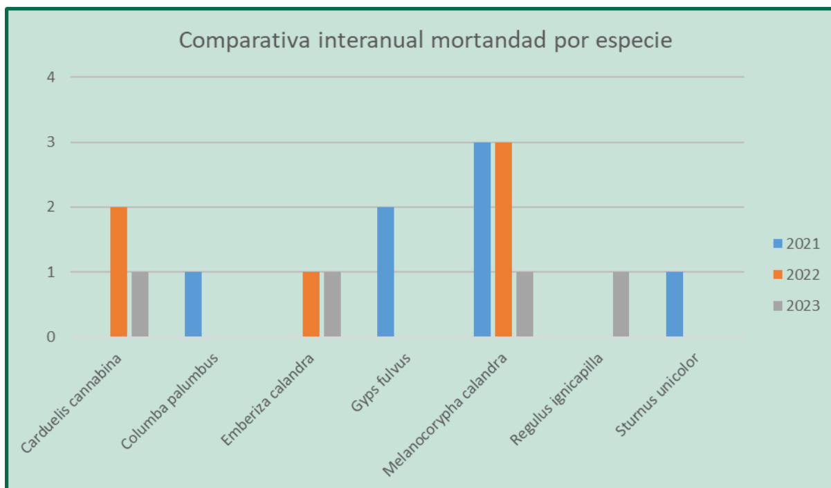
Figura 32. Mortalidad interanual para el primer cuatrimestre por especie, en el PE Las Majas VII E.
