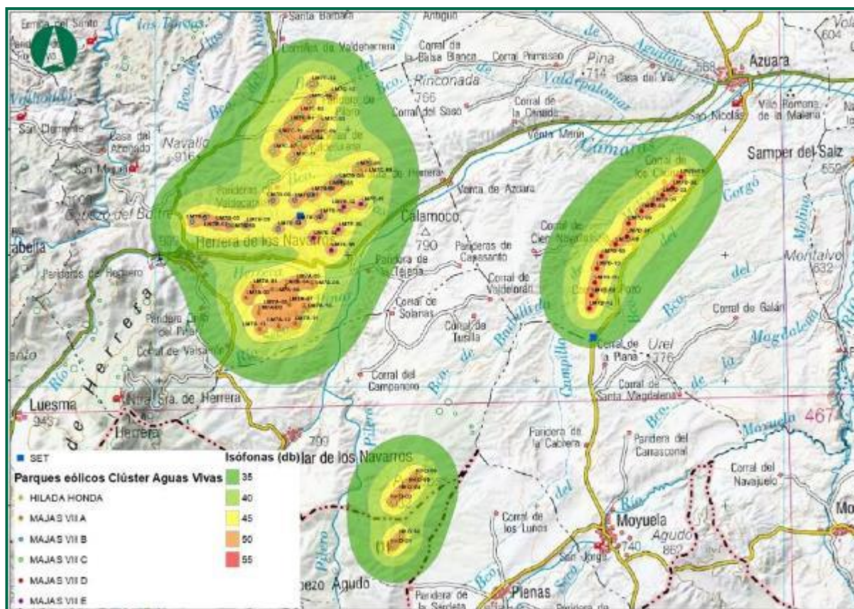
Figura 70. Niveles de presión sonora obtenidos.
