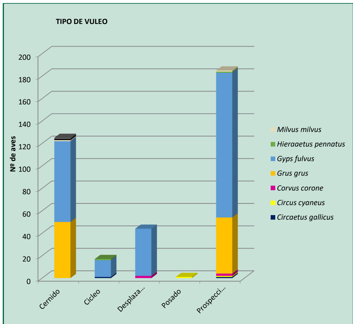
Figura 5. Tipo de vuelos del riesgo por alturas, y especies.
