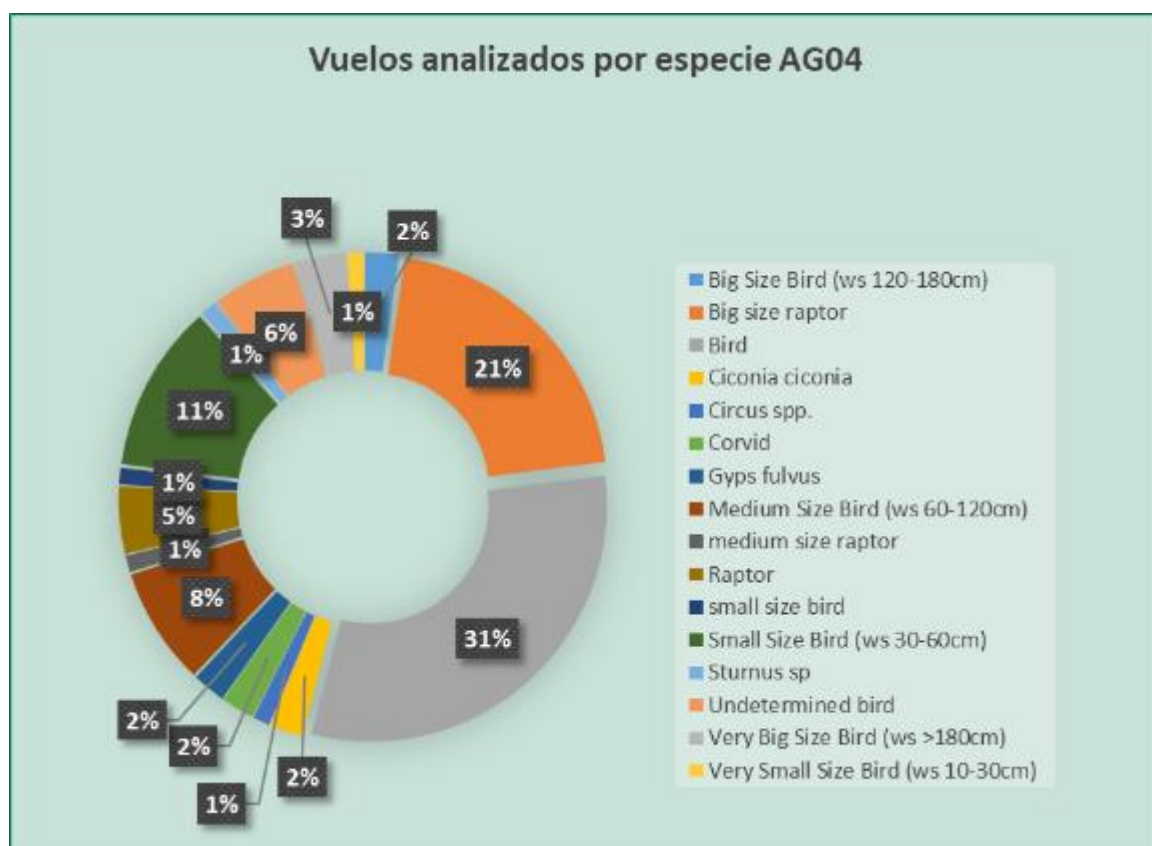
Figura 59. Porcentaje de vuelos por especie/grupo AG04.
