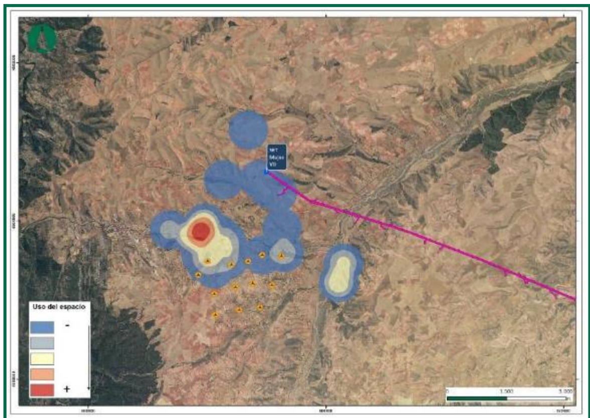
Figura 13. Intensidad del uso del espacio de buitre leonado ( Gyps fulvus ), 1 er cuatrimestre 2023.
