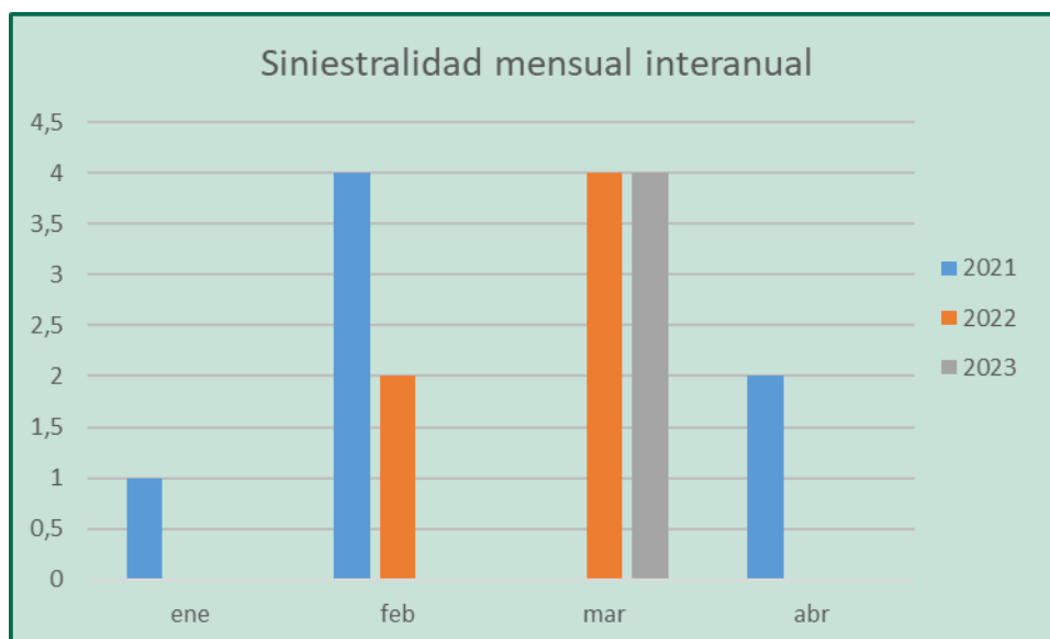
Figura 34. Mortalidad interanual para el primer cuatrimestre por mes, en el PE Las Majas VII E.
