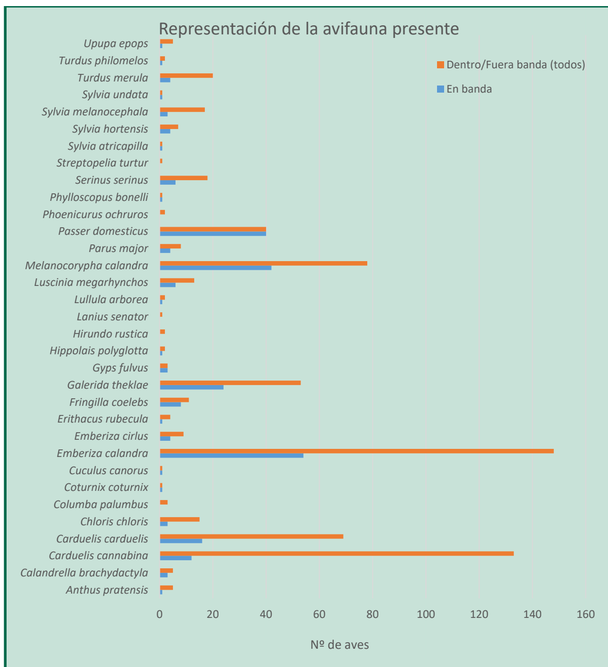
Figura 4. Número de individuos de cada especie observadas.
