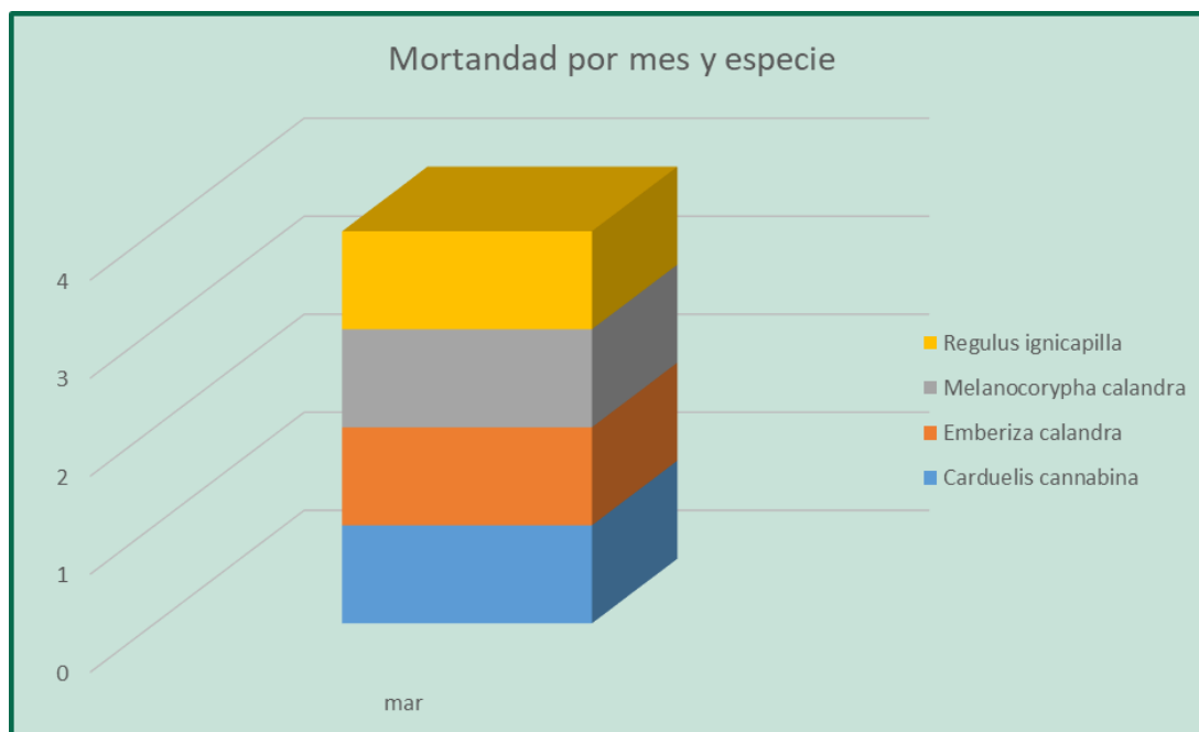
Figura 52. Mortalidad registrada por mes, para el periodo en estudio en el PE Las Majas7E.
