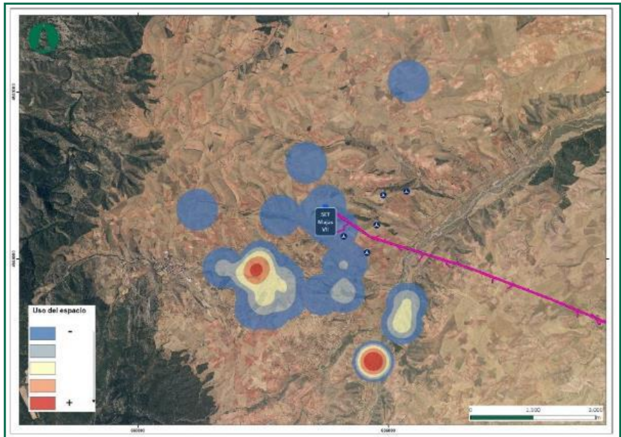
Figura 10. Intensidad del uso del espacio por las aves de gran envergadura detectadas.
