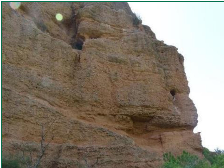
Fotografía 8. Lugar de nidificación de Alimoche ( Neophron percnopterus ) 2022.
