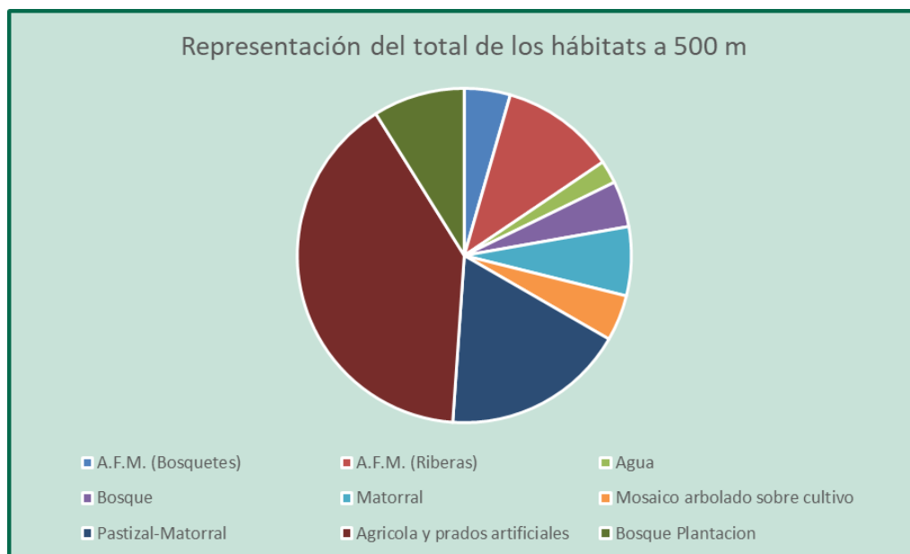
Figura 25. Porcentaje de los hábitats que abarca las estaciones a 500 m.
