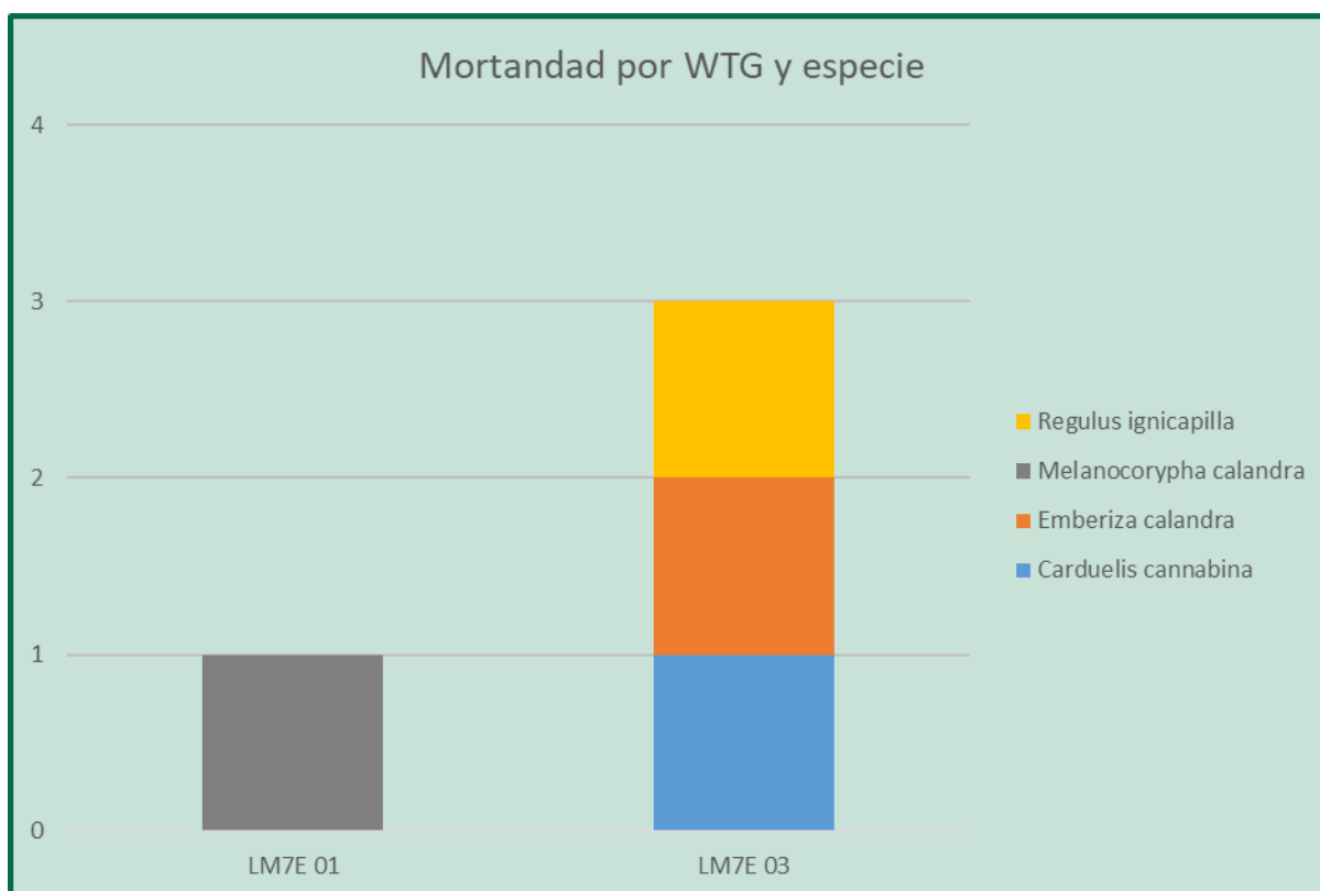
Figura 52. Mortalidad registrada por WTG, para el periodo en estudio en el PE Las Majas7E.
