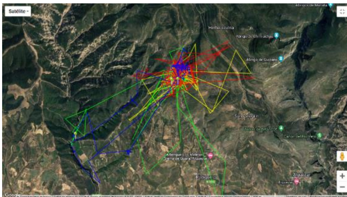
Figura 44. Dispersión de los ejemplares liberados en 2021 durante los primeros días.
