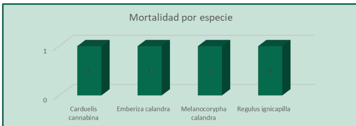
Figura 51. Mortalidad registrada por aerogenerador para el periodo en estudio en el PE Las Majas7E.
