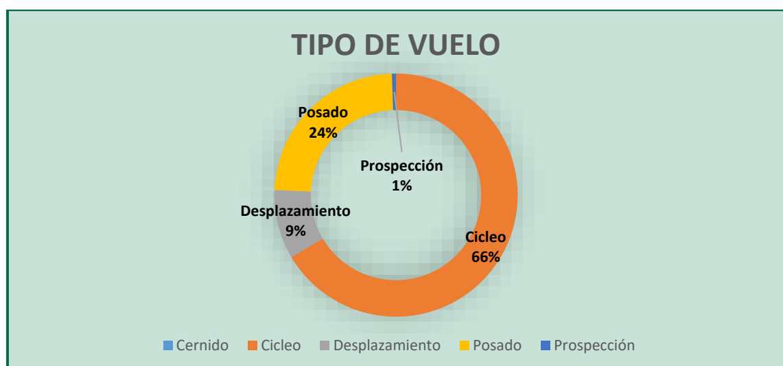
Figura 6. Tipo de vuelos del riesgo por alturas, y especies.
