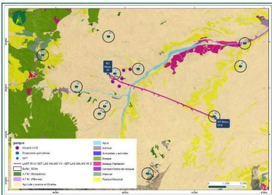
Figura 24. Hábitats en el área de detección en las estaciones de grabación de quiroptero fauna.
