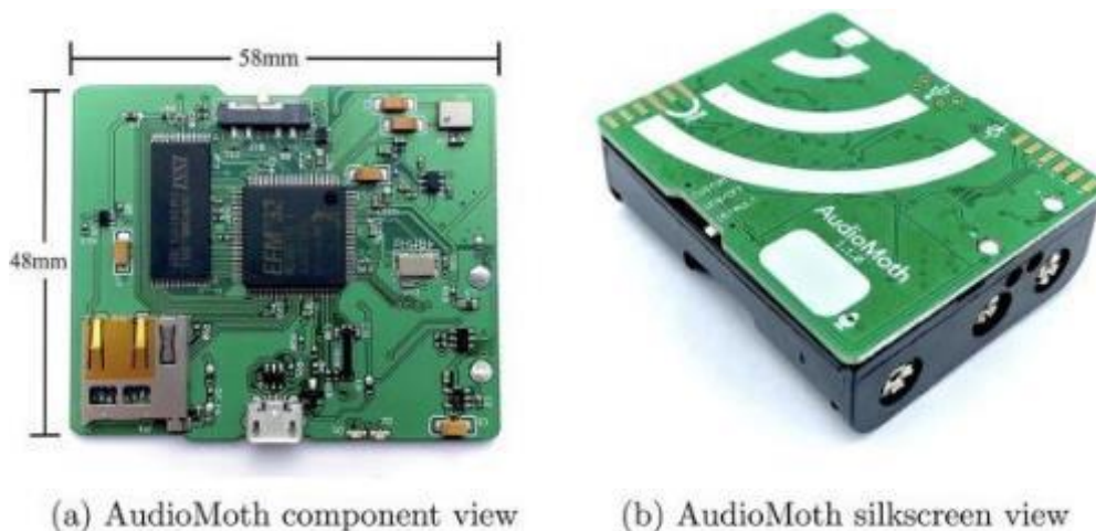
Figura 24. Audiomoth: vista del interior (a) y del exterior (b). Fuente: Hill et al. (2019).
