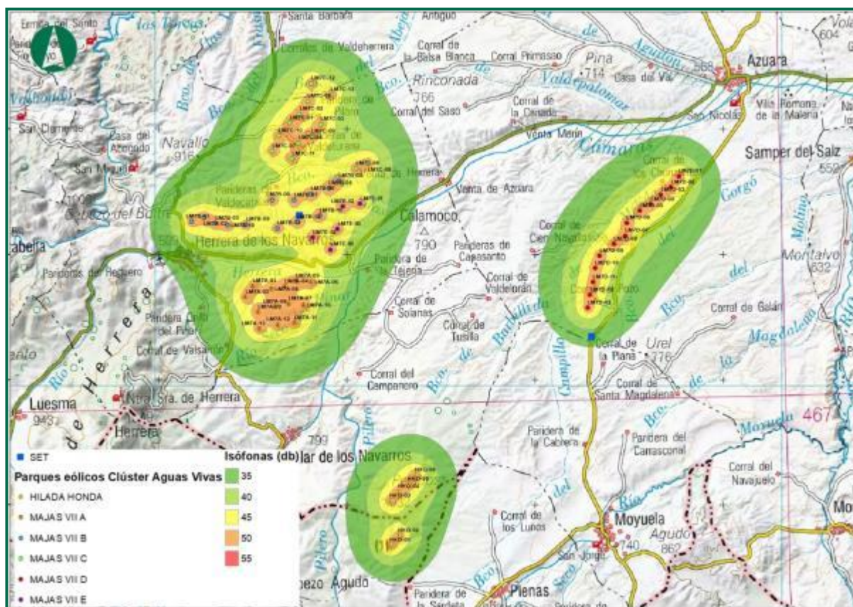
Figura 72. Niveles de presión sonora obtenidos.
