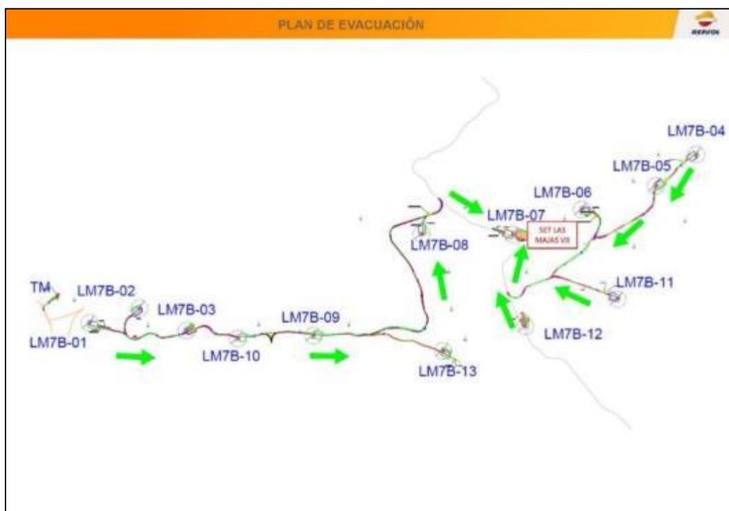
Figura 37. Señalizaciones salidas de evacuación del PE "LM7B".
