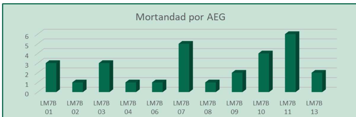
Figura 56. Mortalidad anual por posición, en el PE Las Majas VII B.
