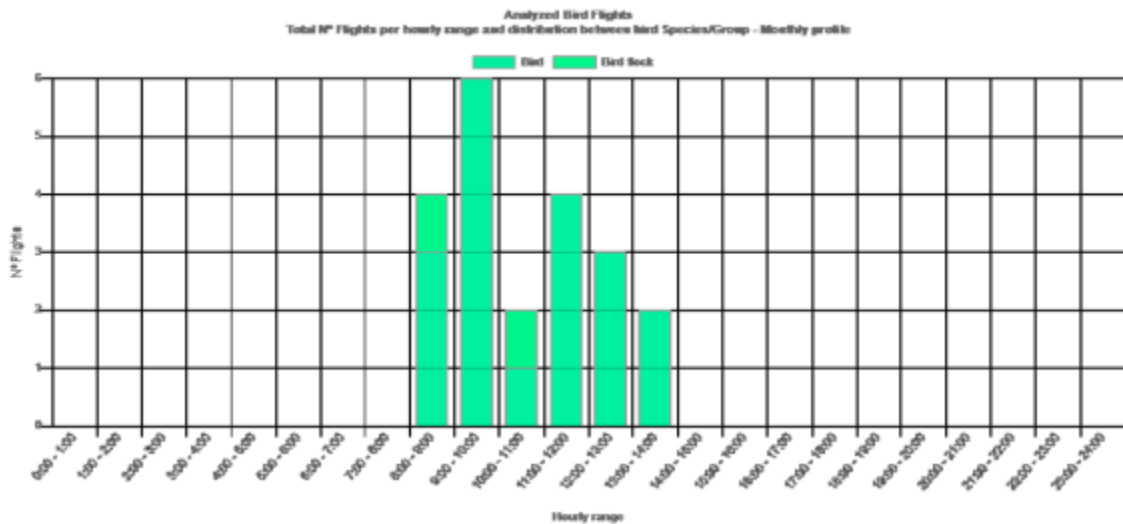
Figura 63. Vuelos analizados por especie, perfil cuatrimestral por horas. WTG LM7B-02 Fuente: DtBird.
