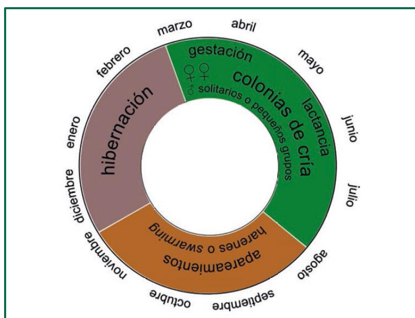
Figura 33. Ciclo biológico anual típico de los murciélagos de zonas templadas. Las fechas que delimitan los diferentes periodos varían dependiendo de la climatología de cada región.
