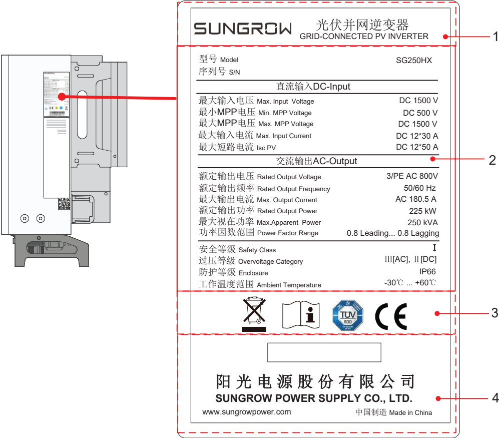
Fig.1. Nameplate
