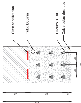
ZANJA N3 - TIPO 2
