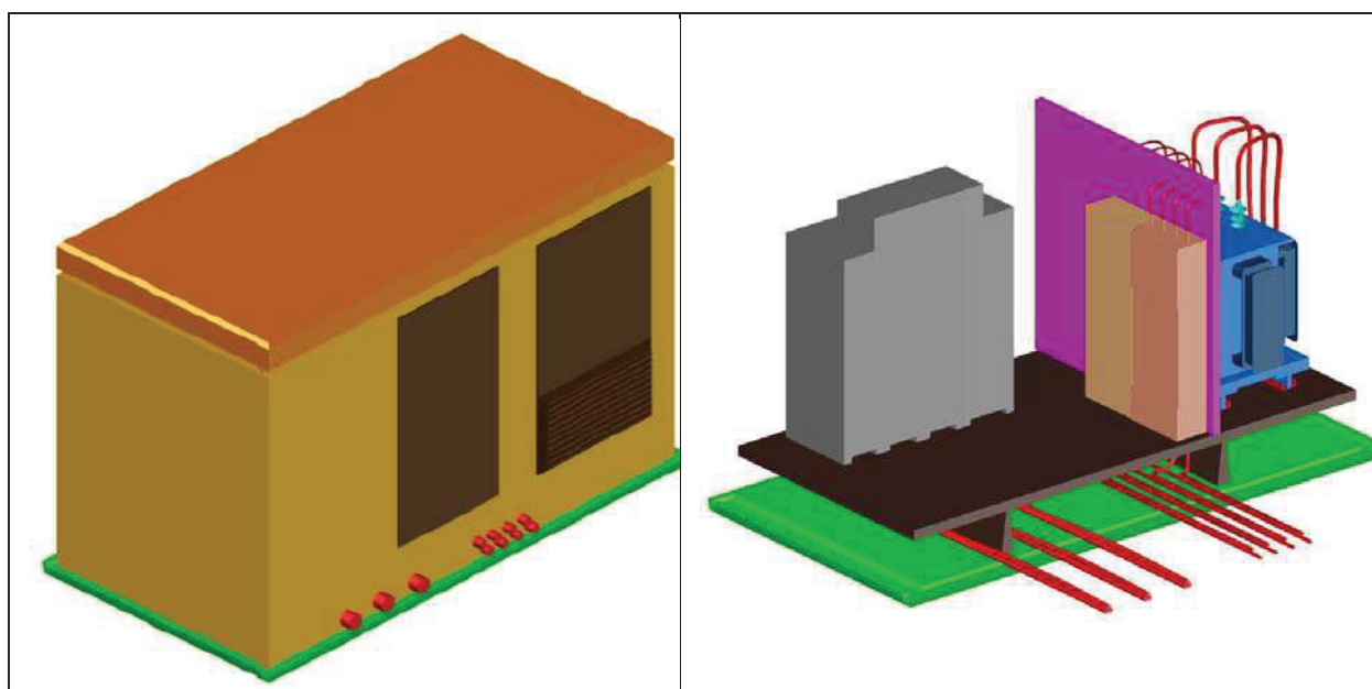
Fig. 1: Vistas 3D Centro transformación tipo en edificio prefabricado de superficie, 24 kV. un trafa.
