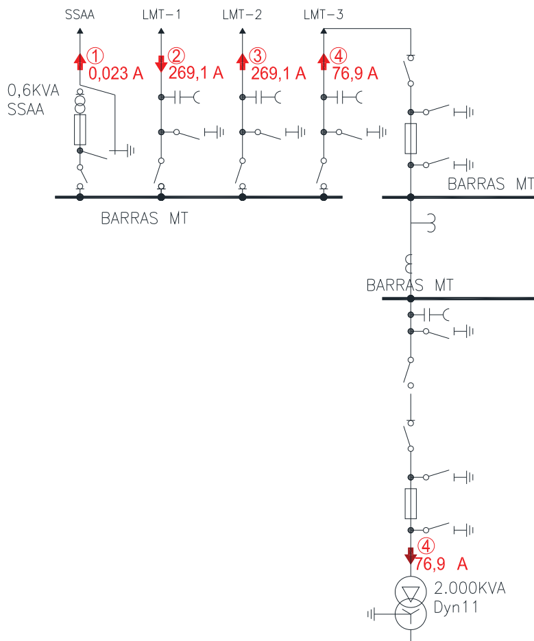
Unifilar nivel de tensión 15kV con intensidades consideradas
