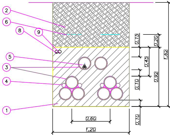
ZANJA PARA DOS CIRCUITOS ALTA TENSIÓN Y DOS CIRCUITOS MEDIA TENSIÓN EN TERRIZO
