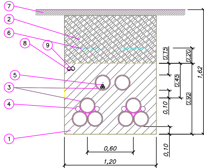
ZANJA PARA DOS CIRCUITOS ALTA TENSIÓN Y DOS CIRCUITOS MEDIA TENSIÓN EN CALZADA
