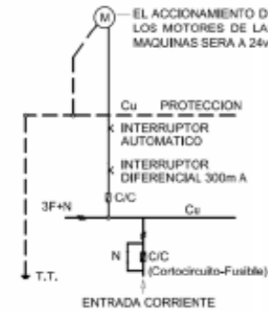
PROTECCION INSTALACION ELECTRICA (ESQUEMA)
