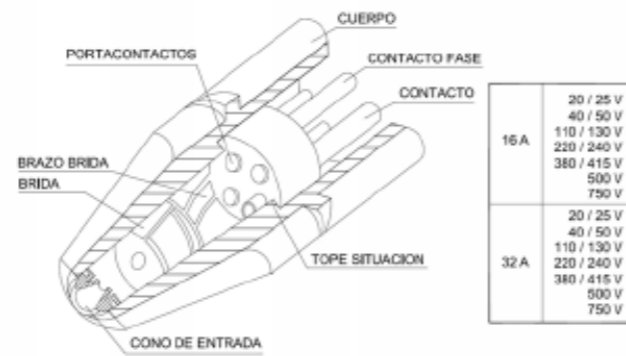
PROLONGADOR TOMA CORRIENTE (CLAVIJA)
