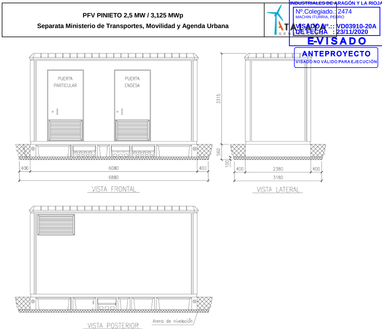
Ilustración 9. Centro de Seccionamiento. Modelo PFU-4. Fuente: Ormazabal
