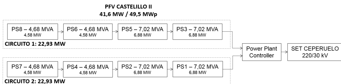
Ilustración 6: Esquema de conexión de la red de MT del PFV
