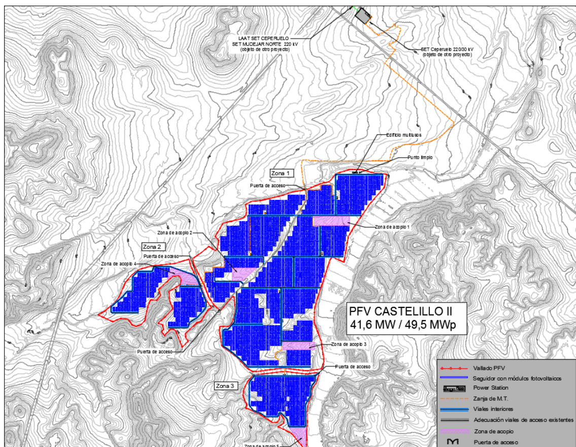
Ilustración 3: Planta general PFV
