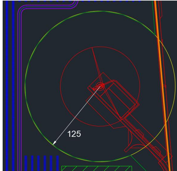
Fig.8 Servidumbre aerogeneradores
