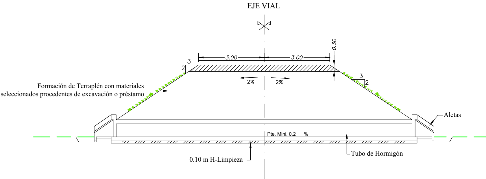
SECCIÓN TIPO VIAL EN TERRAPLÉN (SECCIÓN TIPO CON O.D.) ALETAS-ALETAS
