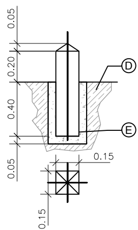
HITO DE SEÑALIZACIÓN DE HORMIGÓN
