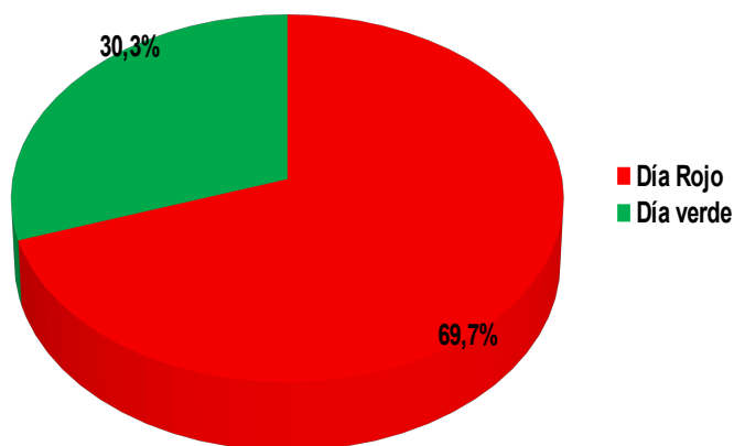
Figura 10.- Porcentaje superficie quemada por tipo de día en las cinco campañas hasta el 31/03/2019.
