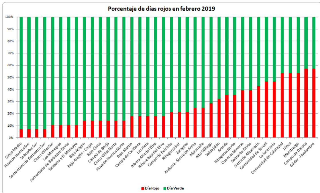
Figura 7.- Índice de Riesgo por Uso del Fuego por comarcas (01/02/2019 – 28/02/2019).
