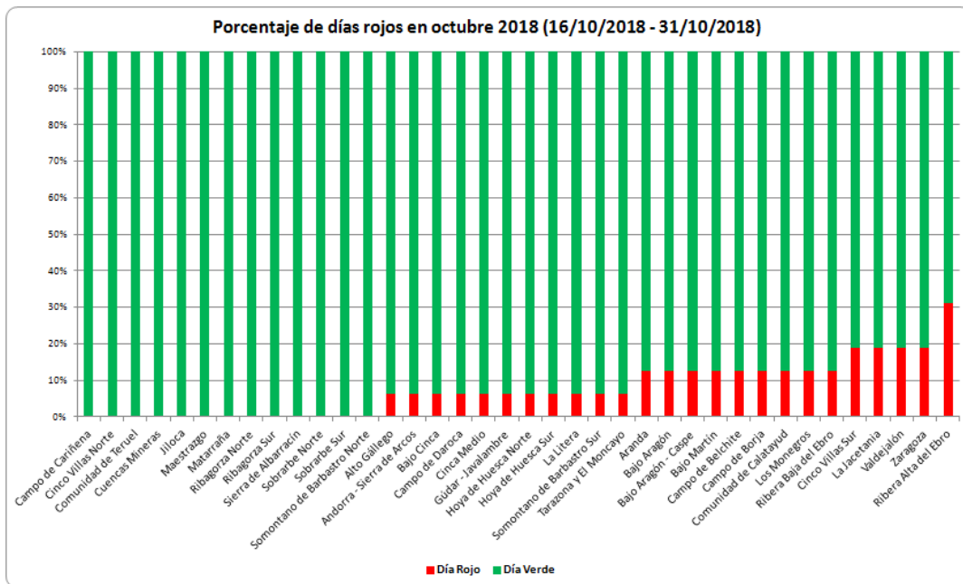
ura 3.- Índice de Riesgo por Uso del Fuego por comarcas (16/10/2018 – 31/10/2018).
