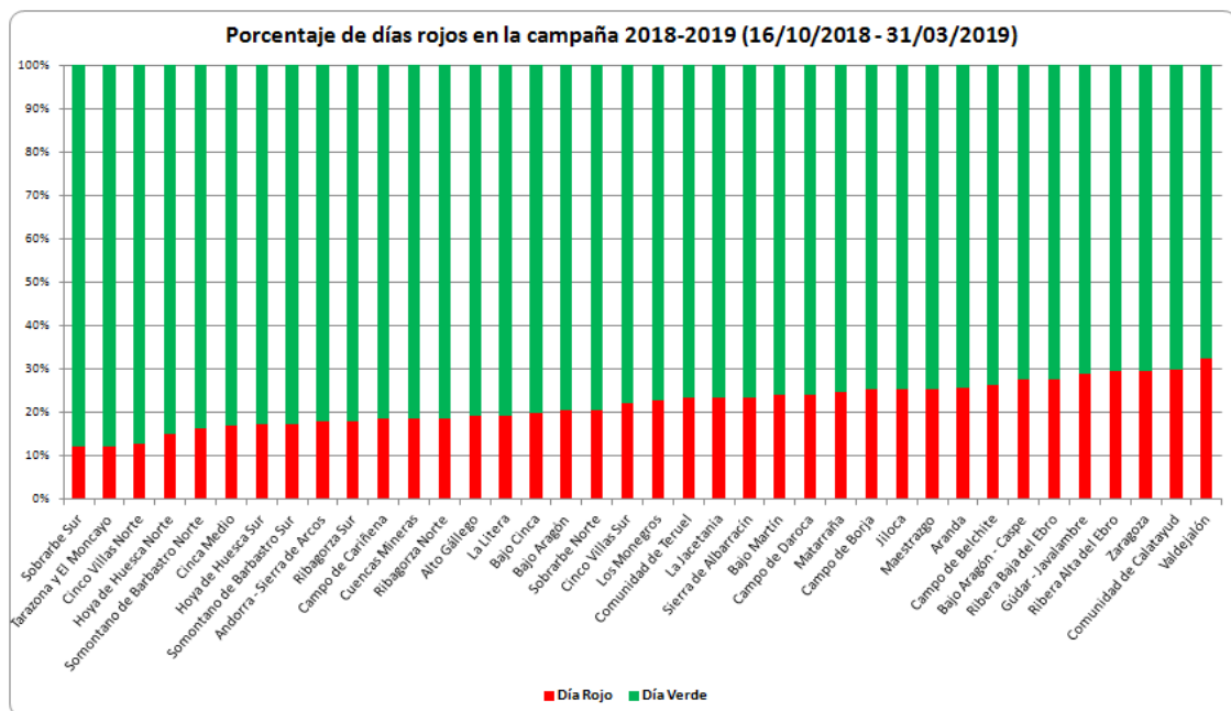
Figura 2.- Índice de Riesgo por Uso del Fuego por comarcas (16/10/2018 – 31/03/2019).
