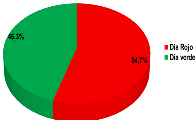
Figura 9.- Porcentaje del número de incendios por tipo de día en las cinco campañas hasta el 31/03/2019.
