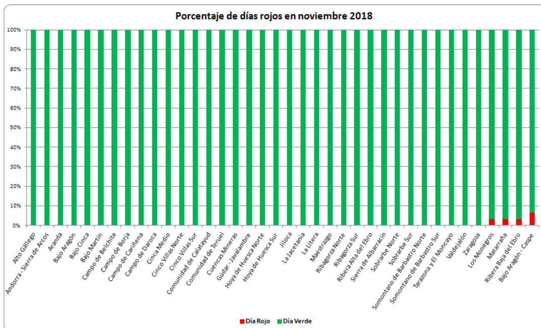
Figura 4.- Índice de Riesgo por Uso del Fuego por comarcas (01/11/2018 – 30/11/2018).
