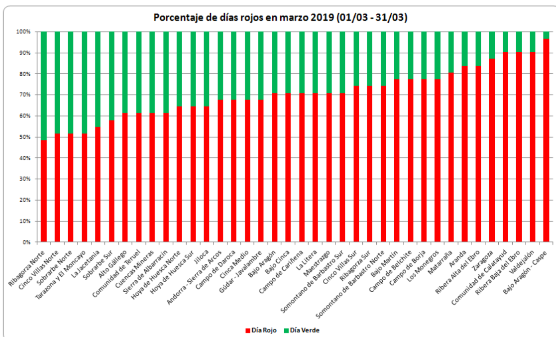
Figura 8.- Índice de Riesgo por Uso del Fuego por comarcas (01/03/2019 – 31/03/2019).
