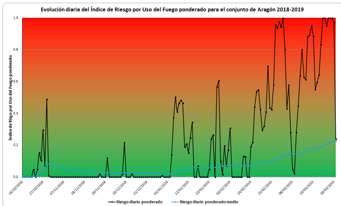
Figura 1.- Índice de Riesgo por Uso del Fuego en Aragón (16/10/2018 – 31/03/2019).
