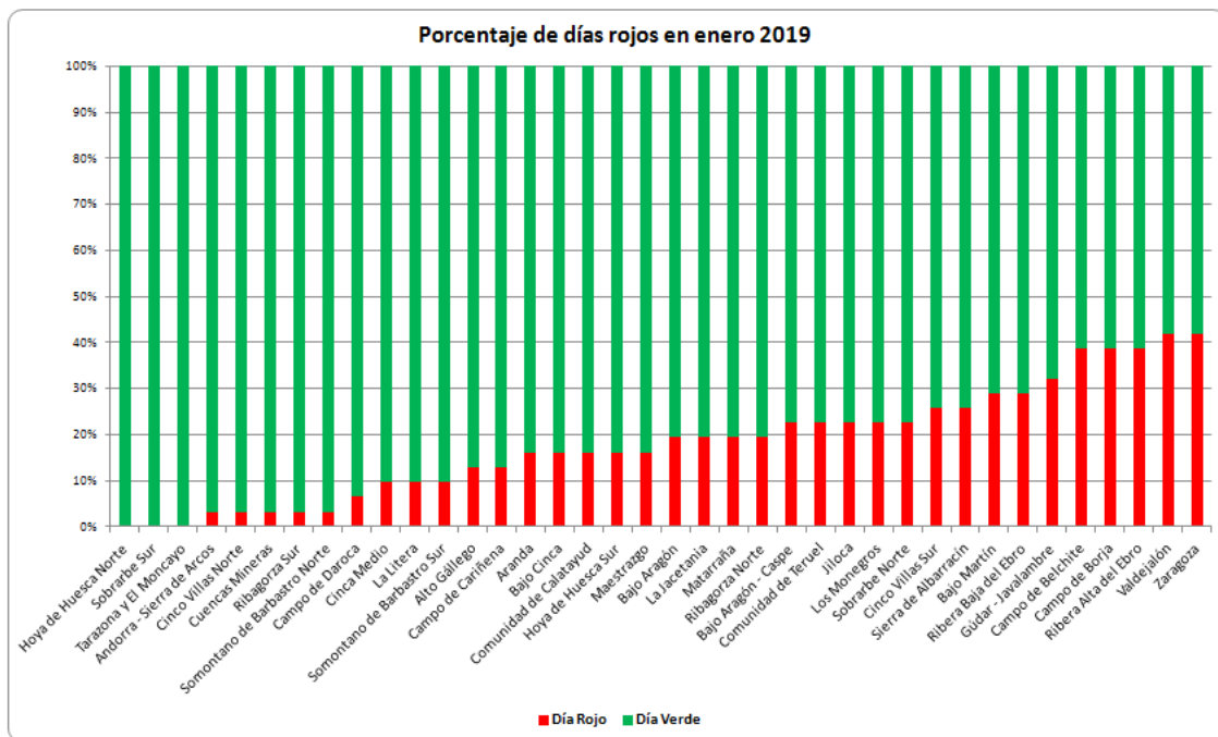
Figura 6.- Índice de Riesgo por Uso del Fuego por comarcas (01/01/2019 – 31/01/2019).
