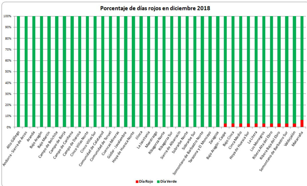
Figura 5.- Índice de Riesgo por Uso del Fuego por comarcas (01/12/2018 – 31/12/2018).
