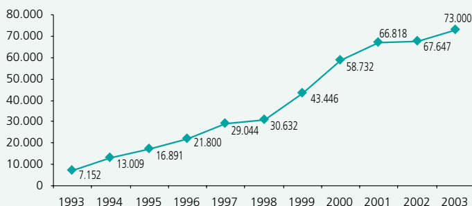
GRÁFICO 55 EVOLUCIÓN DE LA PRODUCCIÓN CONTROLADA DE RESIDUOS PELIGROSOS. ARAGÓN. 1993 A 2003. (TONELADAS)
