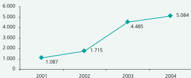
GRÁFICO 54 EVOLUCIÓN DE LA RECOGIDA DE ENVASES LIGEROS. ARAGÓN. 2004 (TONELADAS)
