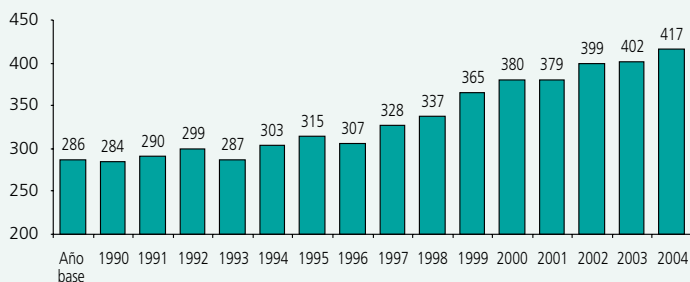
GRÁFICO 52 EMISIONES DE GASES DE INVERNADERO. ESPAÑA. 1990-2004. MILLONES DE TONELADAS DE CO 2 EQUIVALENTE
