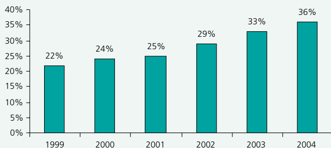
GRÁFICO 53 TASA DE RECUPERACIÓN DE VIDRIO. ARAGÓN. 2004 (PORCENTAJE CON RESPECTO AL VIDRIO CONTENIDO EN LOS RESIDUOS URBANOS)
