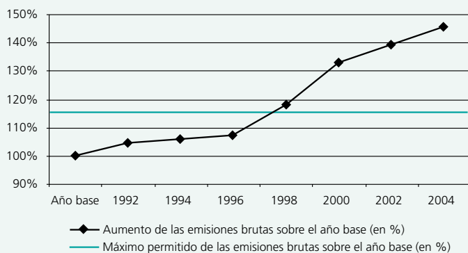
GRÁFICO 51 EVOLUCIÓN DE LAS EMISIONES GEI EN ESPAÑA, EN % SOBRE EL AÑO BASE. 1990-2004
