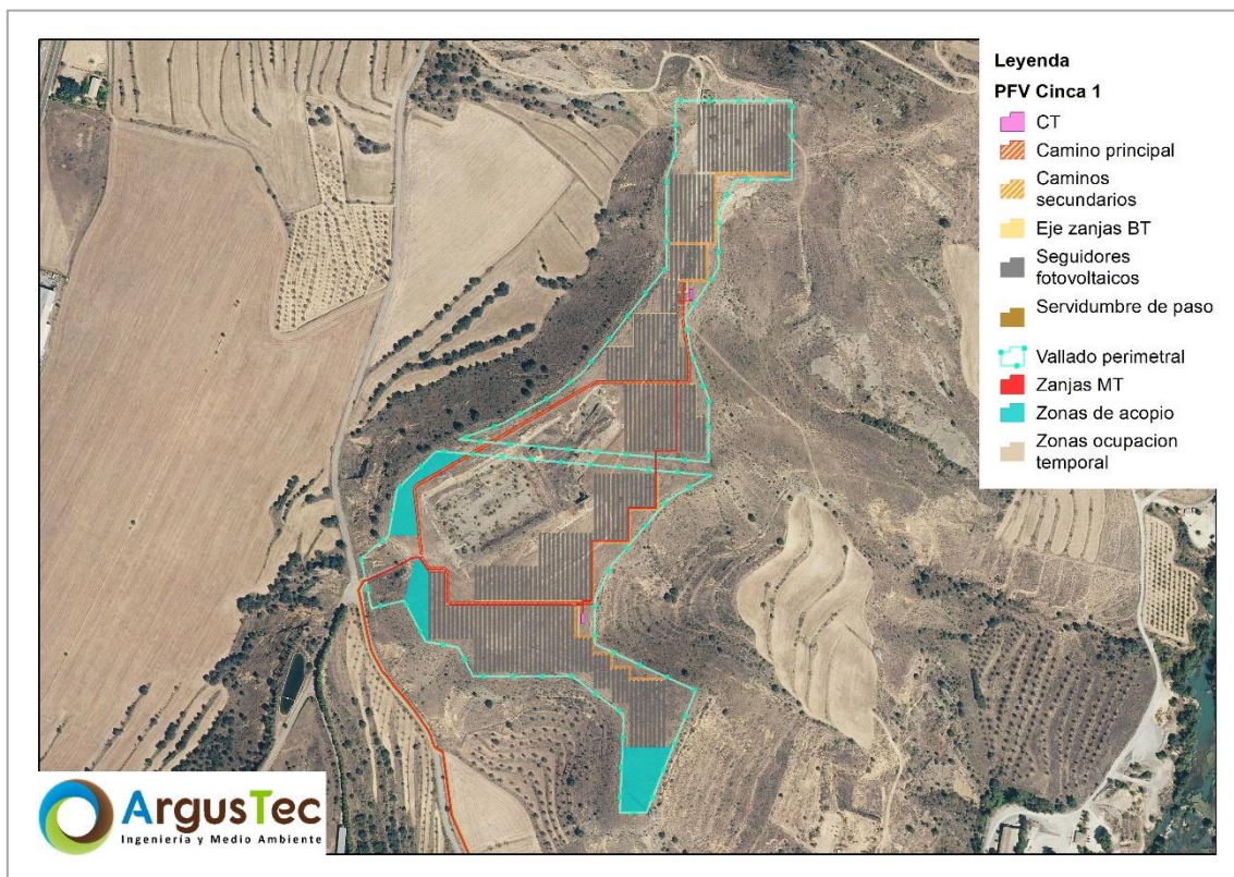
Figura 2. Detalle del parque fotovoltaico Cinca 1
