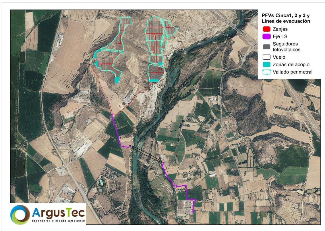
Figura 1. Parques fotovoltaicos y línea de evacuación sobre ortofotografía
