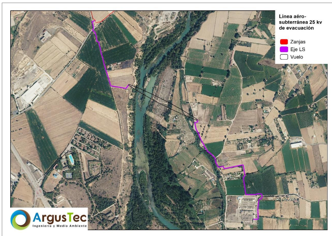
Figura 5. Línea de evacuación común sobre ortofotografía
