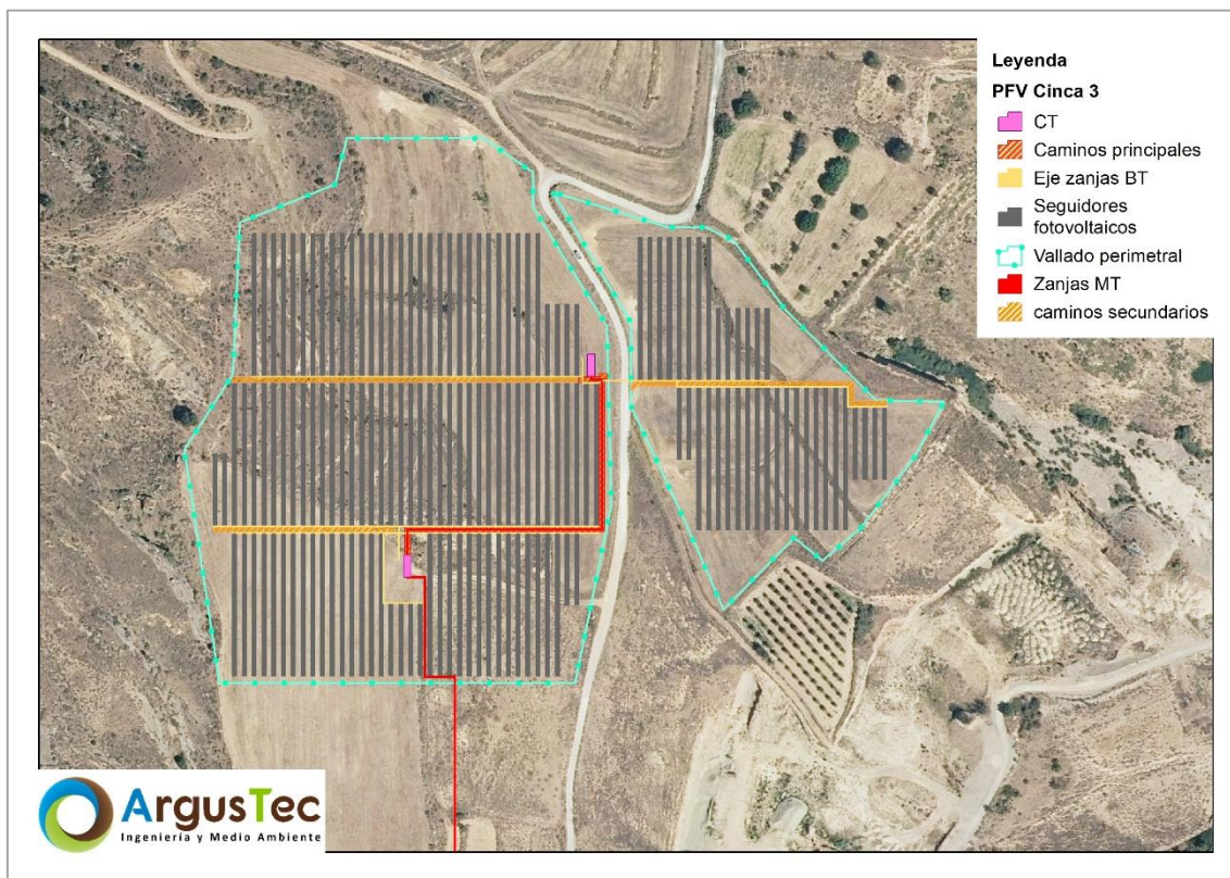
Figura 4. Detalle del parque fotovoltaico Cinca 3
