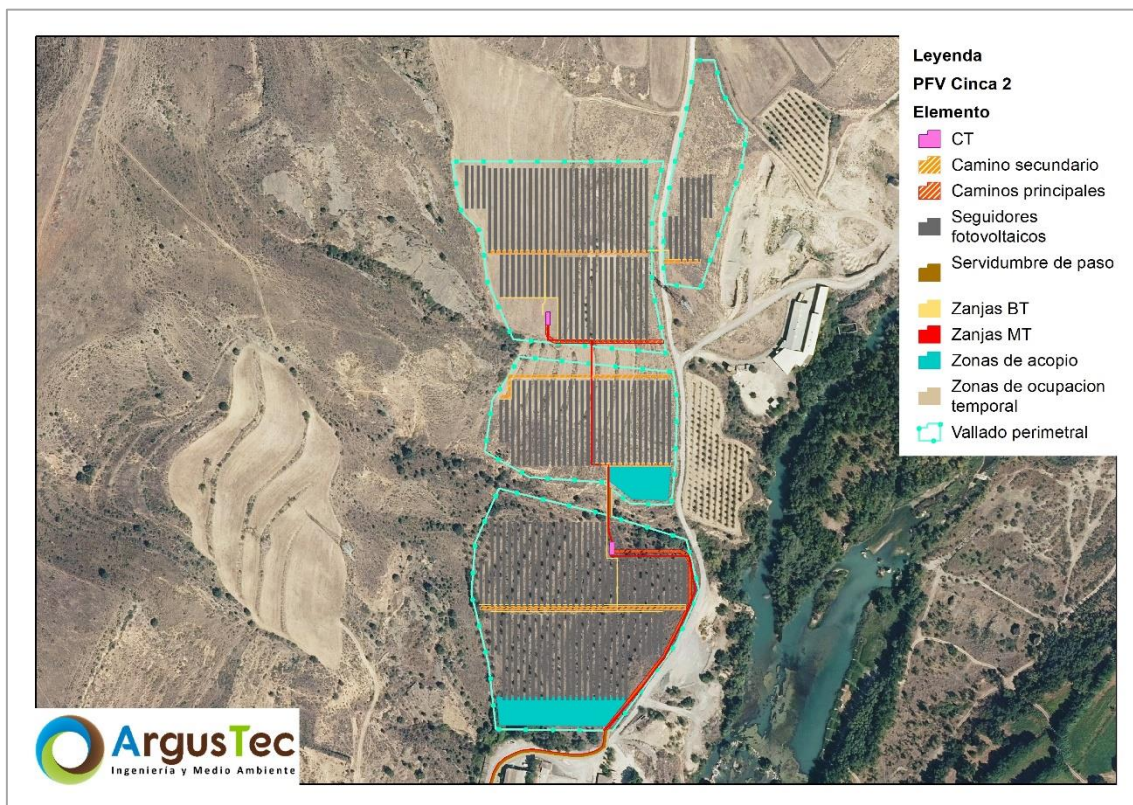
Figura 3. Detalle del parque fotovoltaico Cinca 2
