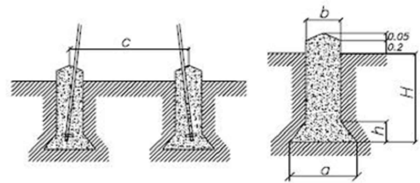
CIMENTACION TETRABLOQUE
