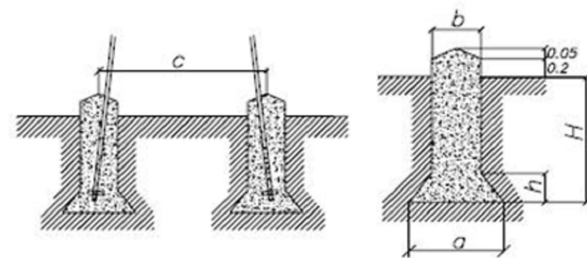
CIMENTACION TETRABLOQUE
