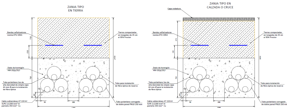
Ilustración 22. Detalle zanja línea subterránea
