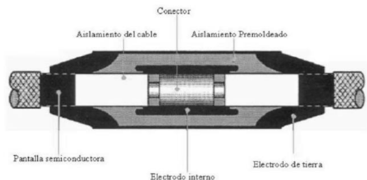
Ilustración 17. Empalmes premoldeados
