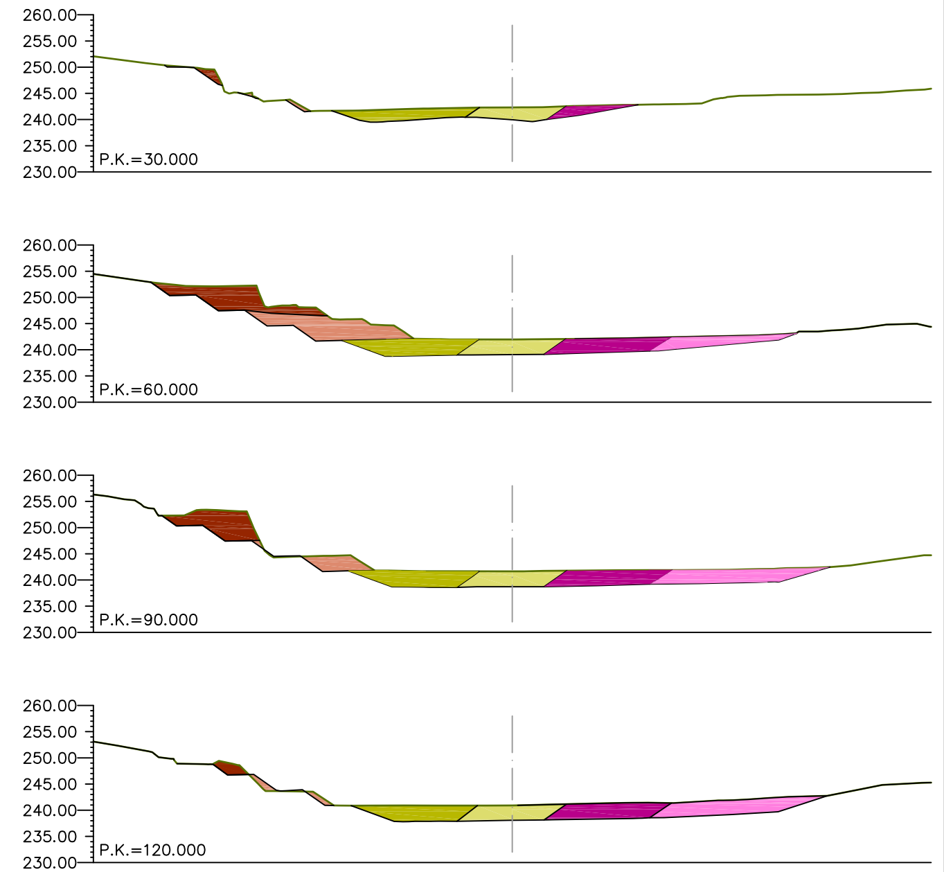
PERFILES TRANSVERSALES. FASES EXPLOTACIÓN
